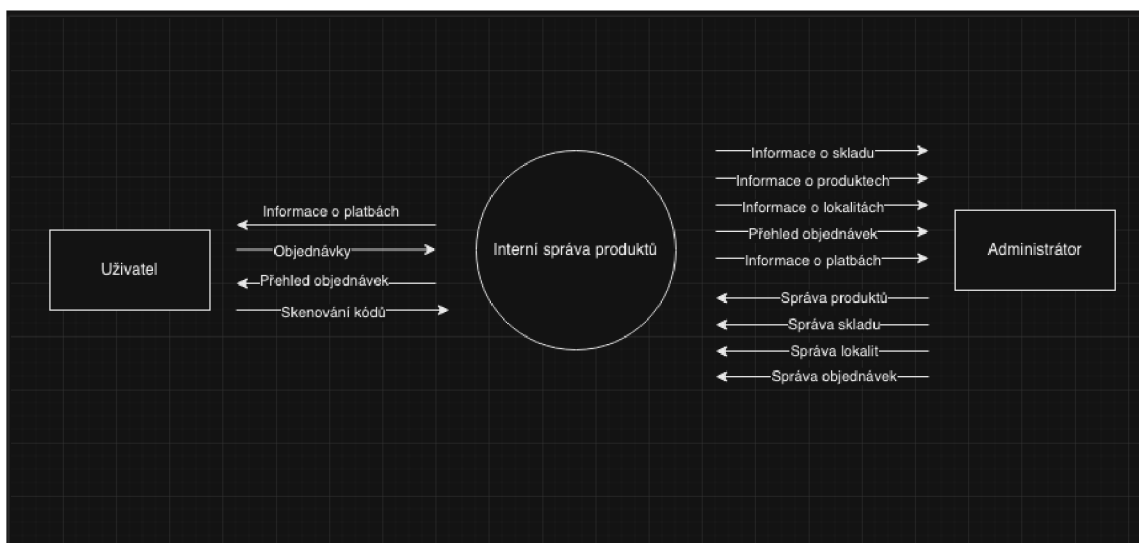
Obrázek 18 DFD diagram systému level 0 (vlastní zdroj)
