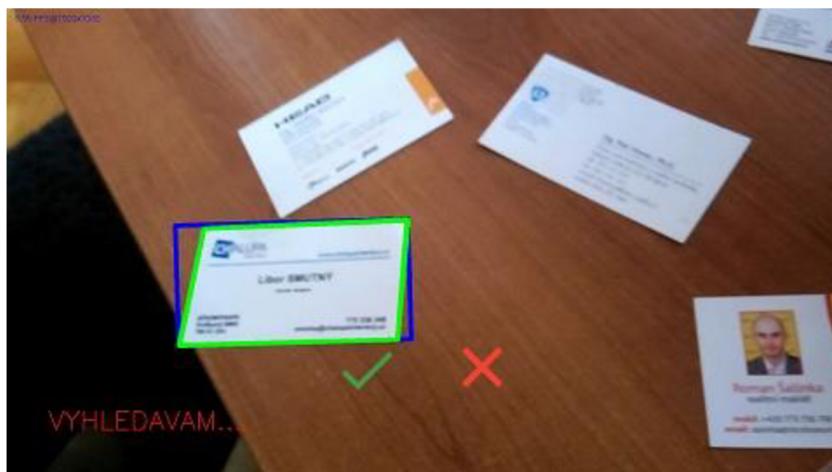
Obrázek 25: Vyhledávání vizitky
