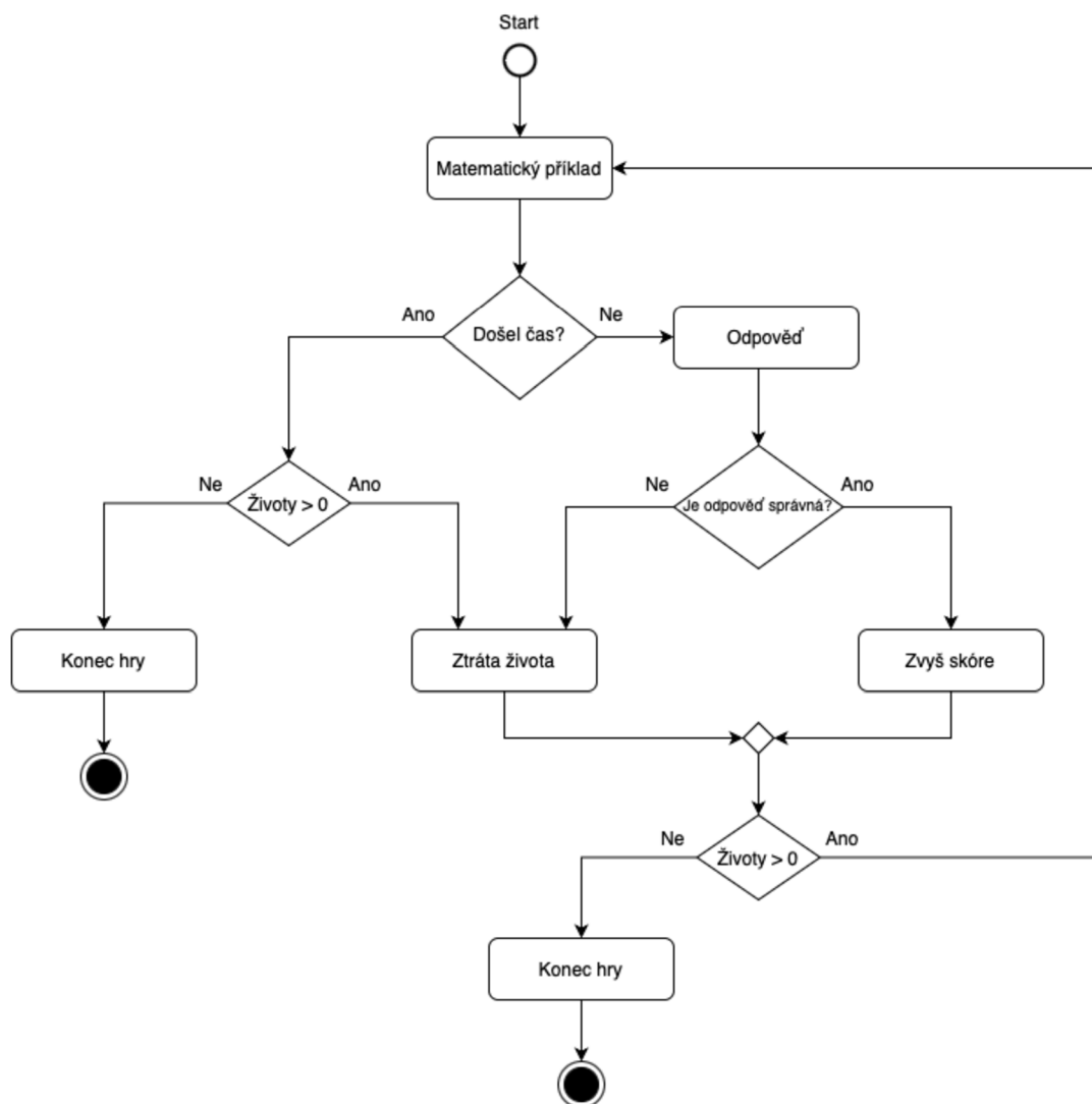
Obrázek 14: Vývojový diagram
