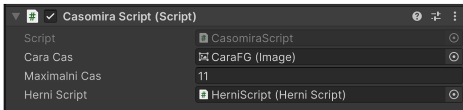
Obrázek 25: Přiřazení proměnných
