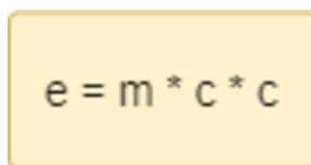
Obrázek 6: Krok algoritmu (34)
