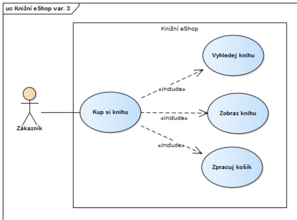
Obrázek 4: Příklad use-diagramu (31)
