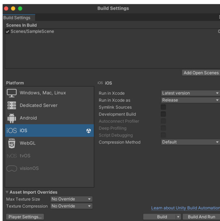
Obrázek 19: Nastavení buildu
