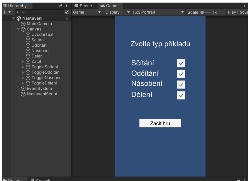
Obrázek 21: Druhá scéna
