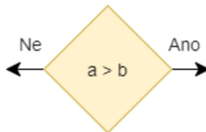
Obrázek 8: Podmínka (34)
