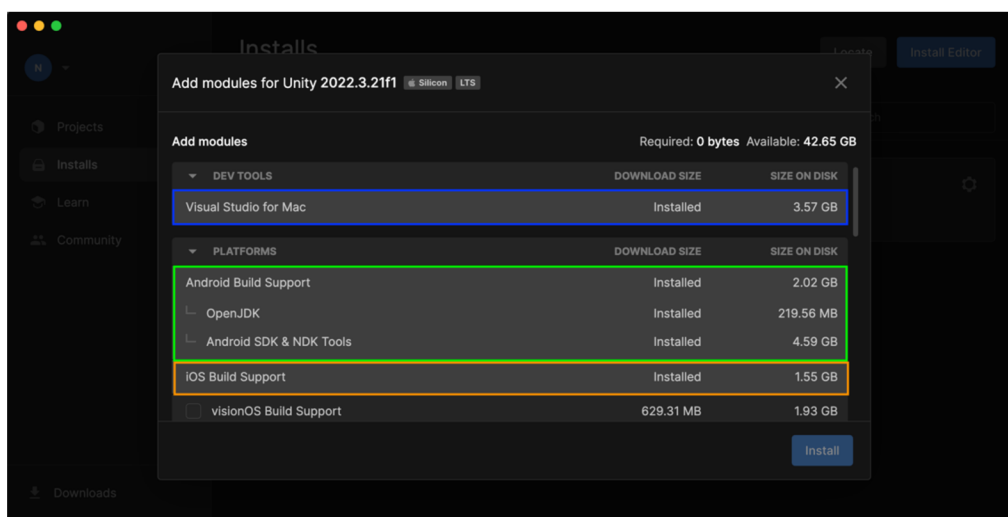
Obrázek 16: Instalace modulů
