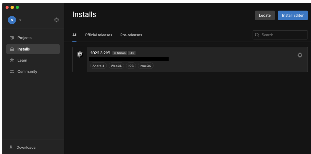
Obrázek 15: Unity hub
