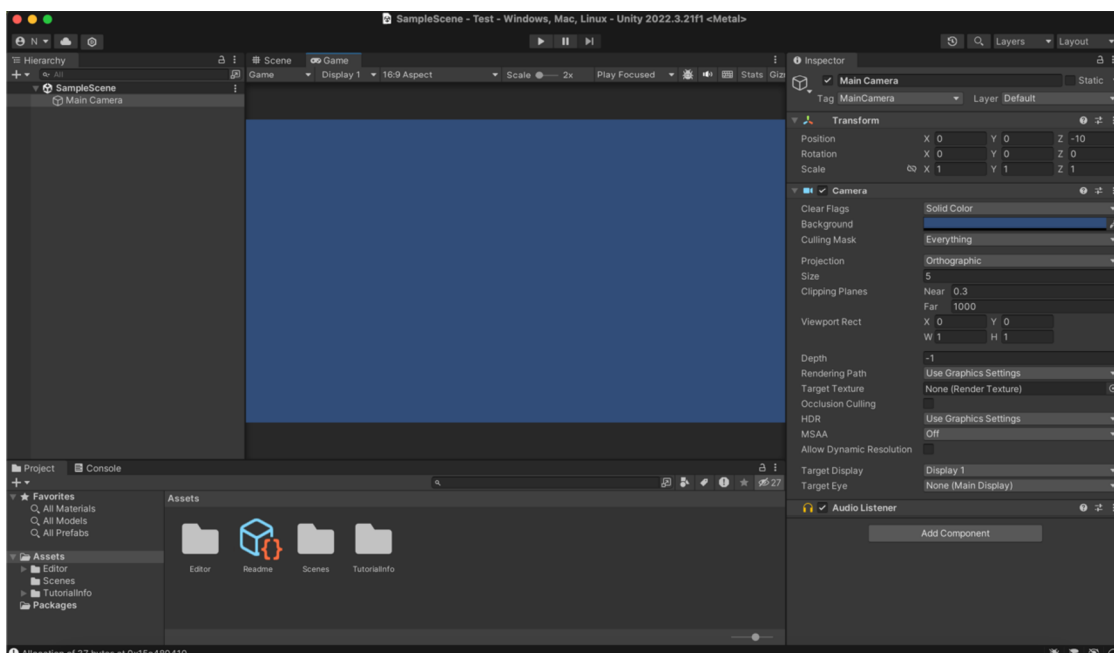
Obrázek 18: Rozhraní unity
