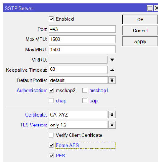
Obrázek 13: Konfigurace SSTP serveru (Zdroj: vlastní zpracování)
