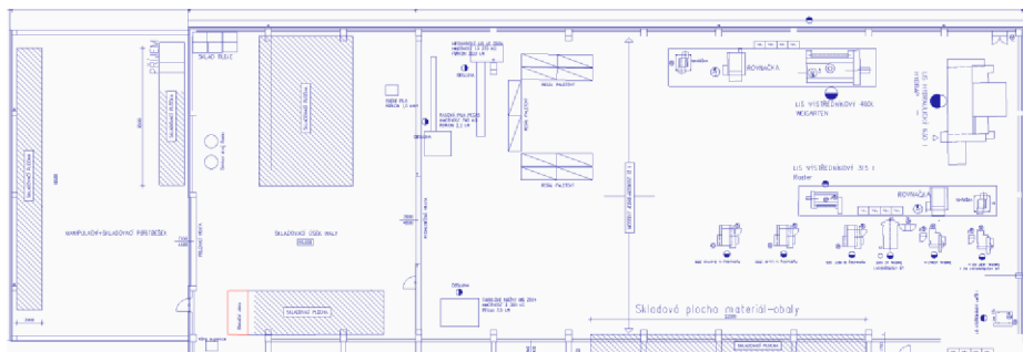
Obrázek 9: Půdorys haly 3 (Zdroj: poskytla společnost)
