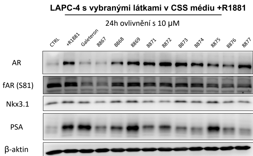
Obr. 16 – Výsledek imunodetekce vybraných proteinů buněčné linie LAPC-4 po ovlivnění vybranými látkami a galeteronem o konečné koncentraci 10 \mu M a době ovlivnění 24 hodin. Ke všem vzorkům, krom vzorku CTRL, byl přidán 1nM R1881. Bylo použito 10% stripované sérum (CSS) DMEM s takřka nulovou bazální hladinou androgenů. AR značí androgenní receptor, fAR (S81) značí fosforylovanou formu AR na serinu v pozici 81, PSA značí prostatický specifický antigen. Detekce \beta -aktinu značí rovnoměrné nanesení vzorku.
