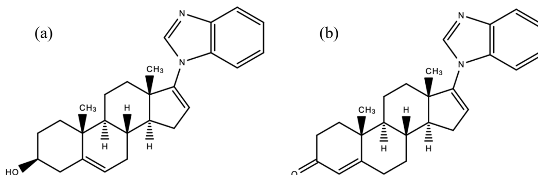
Obr. 5 – (a) Strukturní vzorec galeteronu. (b) Strukturní vzorec \Delta(4) -galeteronu. Shodné kruhy A a B mezi testosteronem a D4G jsou příčinou silného antagonistického charakteru D4G (Alyamani a kol., 2017).
