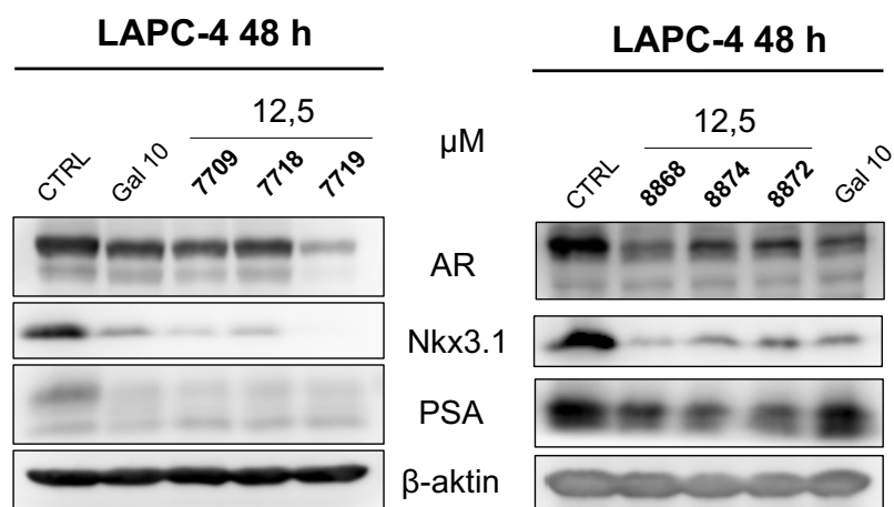
Obr. 18 – Výsledky imunodetekce vybraných proteinů buněčné linie LAPC-4 v plném DMEM médiu po ovlivnění vybranými látkami o konečné koncentraci 12,5 \mu M a galeteronem o konečné koncentraci 10 \mu M (Gal 10) při době ovlivnění 48 hodin. AR značí androgenní receptor a PSA značí prostatický specifický antigen. Detekce \beta -aktinu značí rovnoměrné nanesení vzorku.
