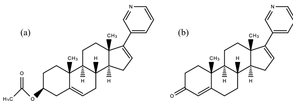
Obr. 4 – (a) Strukturní vzorec abirateron acetátu. (b) Strukturní vzorec \Delta(4) -abirateronu. Shodné kruhy A a B mezi testosteronem a D4A jsou příčinou antagonistického charakteru D4A (Li a kol., 2015).
