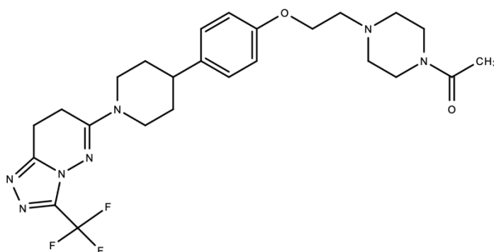
Obr. 9 – Strukturní vzorec AZD3514, antagonisty AR druhé generace, který krom inhibice AR skrze zamezení translokace AR do jádra také snižuje syntézu AR.
