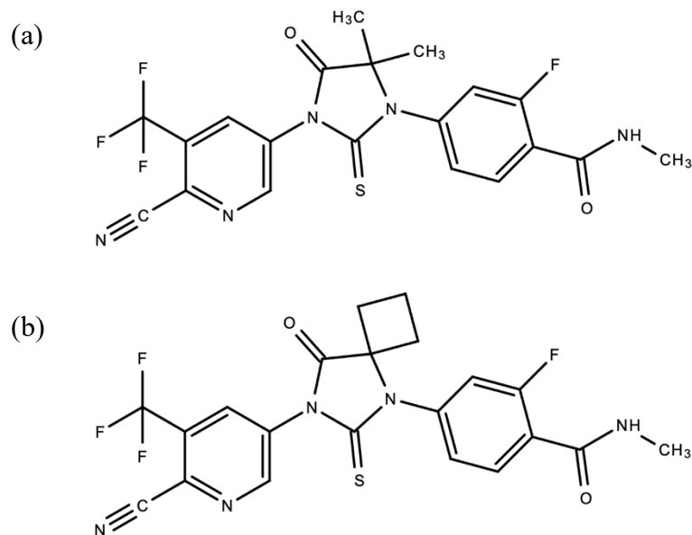
Obr. 8 – Strukturální vzorce dvou významných antagonistů AR druhé generace: (a) apalutamidu a (b) enzalutamidu. Patrná je výrazná strukturální podobnost.
