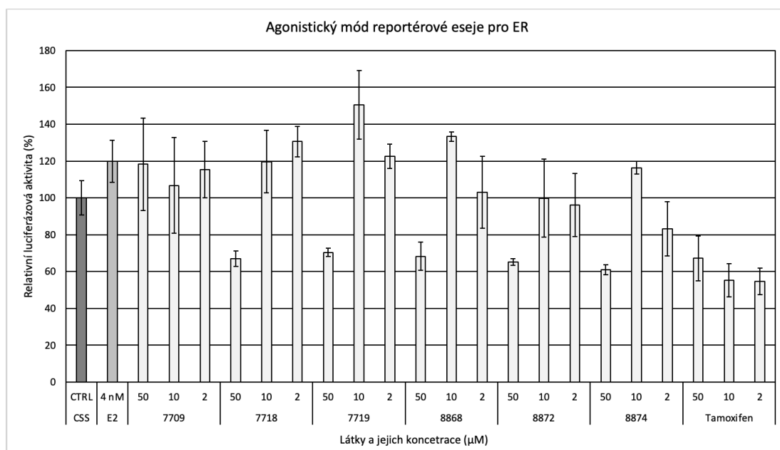
Obr. 28 – Výsledný graf agonistického módu reportérové eseje pro ER. Relativní luciferázová aktivita byla vypočtena poměrem mezi průměrným signálem FNC luciferázy pro daný vzorek ku průměrné hodnotě signálu RNC luciferázy v rámci měřené 96jamkové desky. Tento poměr byl následně normalizován na signál kontroly s prázdnou transfekcí v CSS médiu (100 %).
