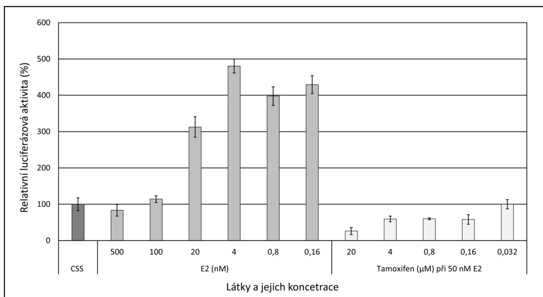
Obr. 27 – Výsledky optimalizační reportérové eseje pro ER. Graf relativní luciferázové aktivity (%) v závislosti na použité koncentraci 17 \beta -estradiol (E2) a tamoxifenu, ke kterému bylo přidáno 50 nM E2. Signál FNC luciferázy u každého vzorku byl vztažen na průměrný signál RNC luciferázy z celého měření.
