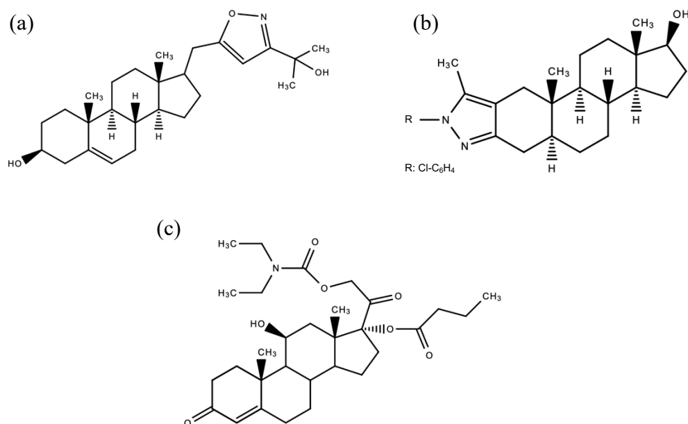
Obr. 7 – Strukturní vzorce látek (a) 24j (Rudovich a kol., 2022), (b) 3d (Peřina a kol., 2023b) a (c) 14 (Peřina a kol., 2023a).
