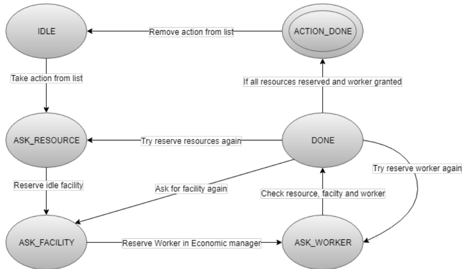
Obrázek 7.2: Stavový automat zajišťující provádění akcí v Infrastructure managerovi
