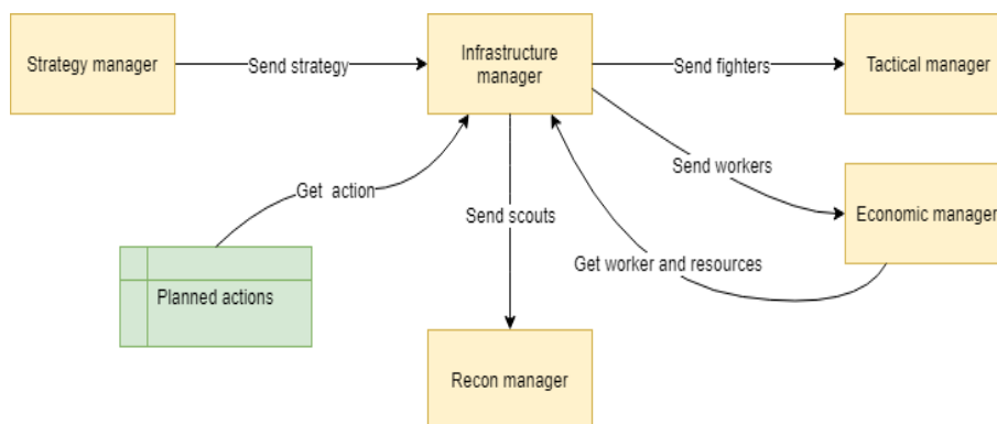
Obrázek 6.3: Schéma Infrastructure managera
