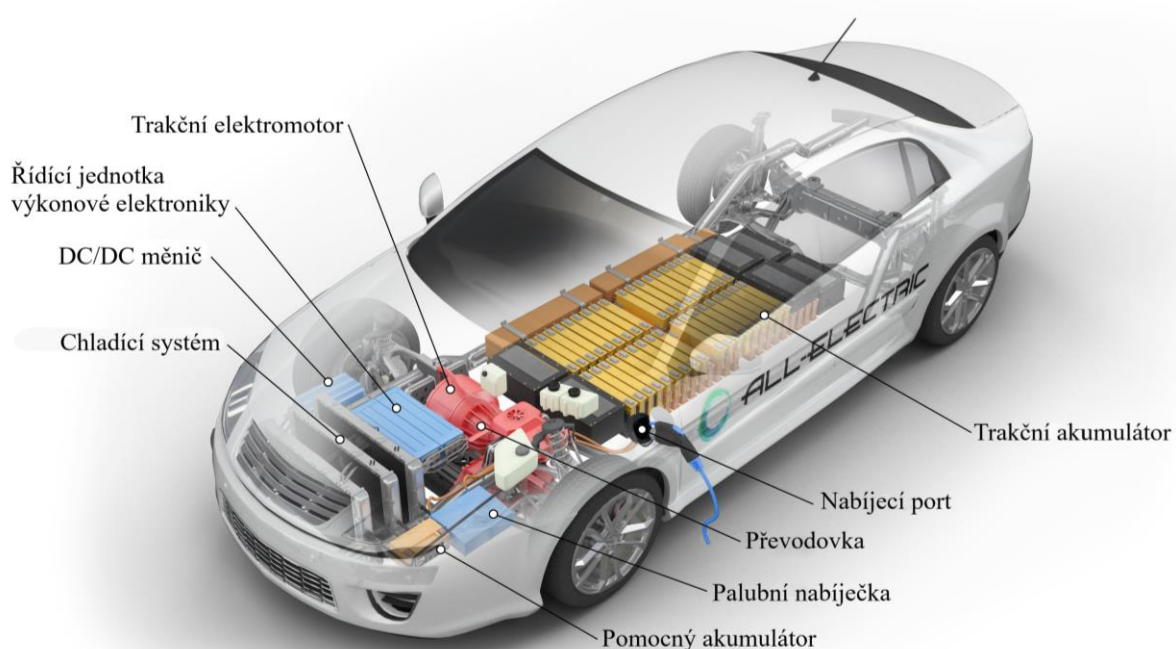
Obr. 2 Hlavní součásti elektromobilu (upraveno)
