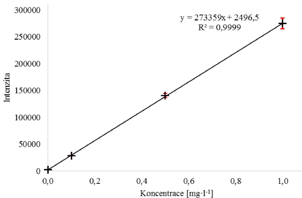
Graf 2 Kalibrační přímka pro stanovení Mn při analýze vzorků č. 1 a 2
