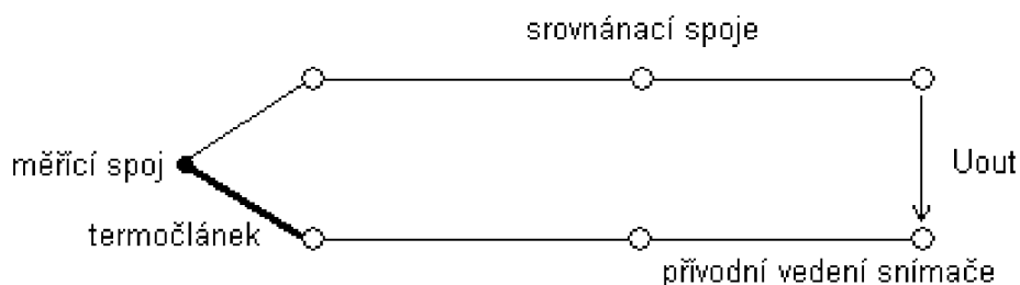
Obr. 3.5: Termočlánek
