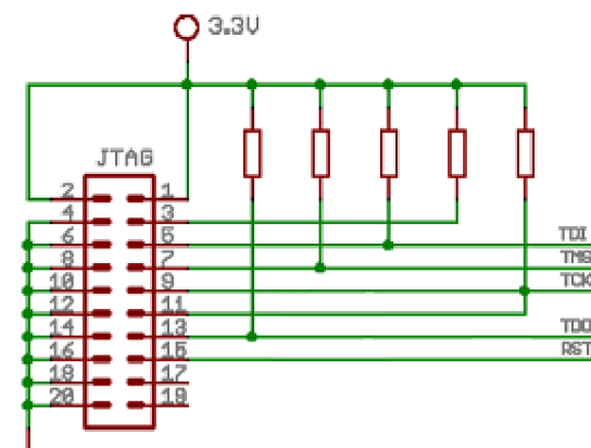
Obr. 5.16: Zapojení rozhraní JTAG včetně standardního 20ti pinového konektoru
