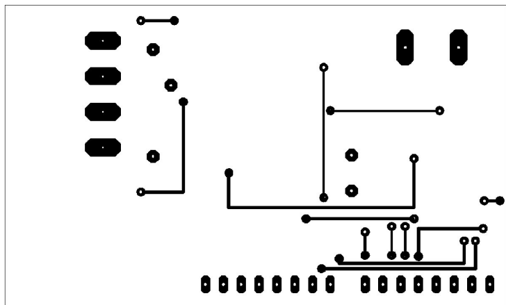
Příloha 0.6: Deska plošných spojů - BOTTOM
