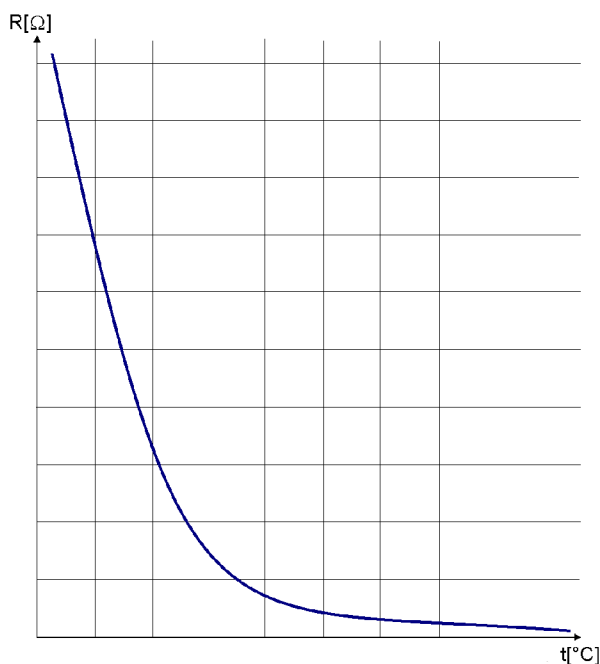
Obr. 3.2: Závislost odporu negastoru na teplotě
