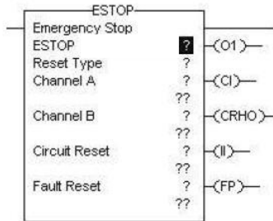
Obr. 6-3 Blok ESTOP [24].
