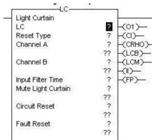
Obr. 6-2 Blok LC [24].
