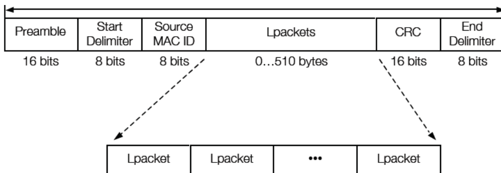
Obr. 2-10 MAC rámec ControlNet [2].
