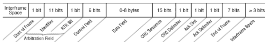
Obr. 2-6 CAN komunikační paket [5].
