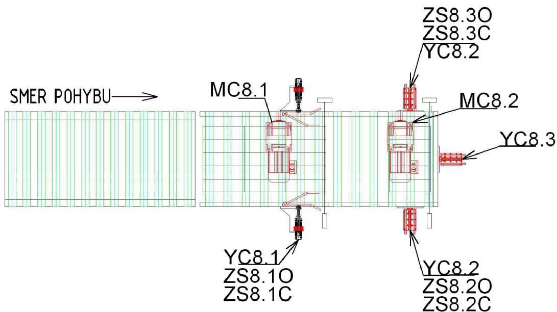
Obr. 2.10: Schéma odebíracích dopravníků balíků
