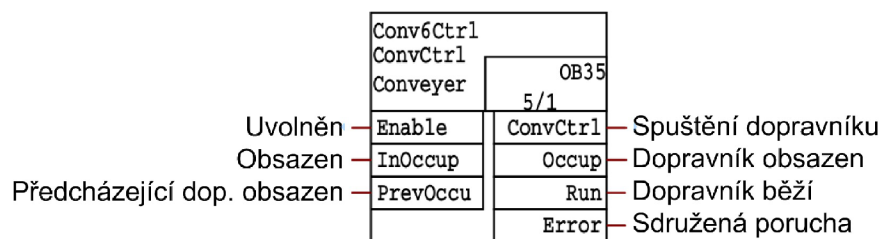
Obr. 8.11: CFC odebíracího dopravníku 6
