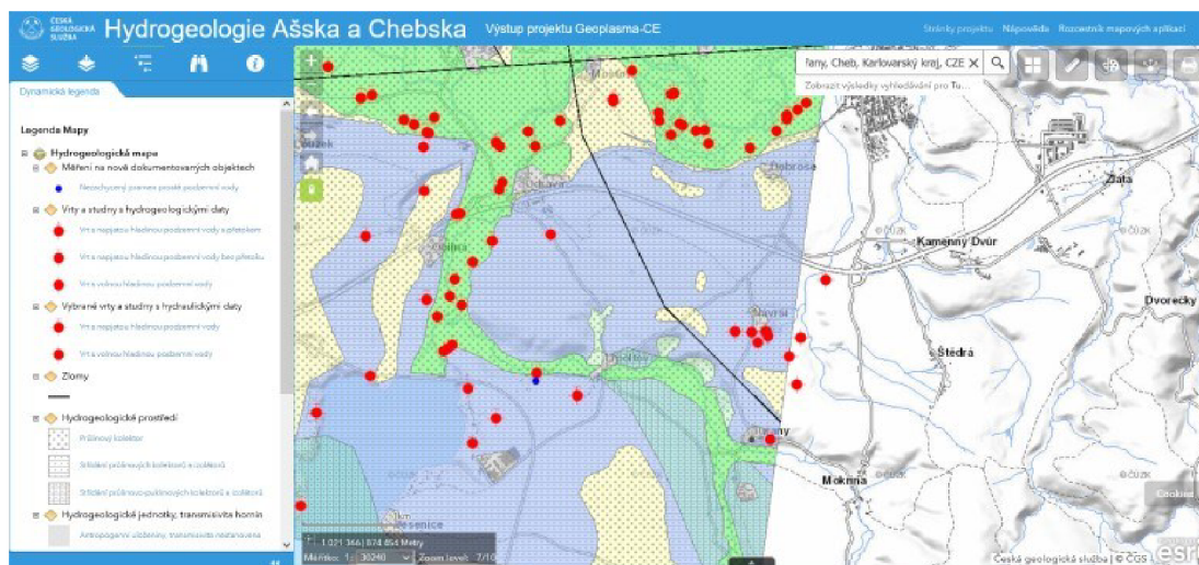
Obr. 15: Hydrogeologická mapka k. ú. Tuřany (ČGS, © 2023)
