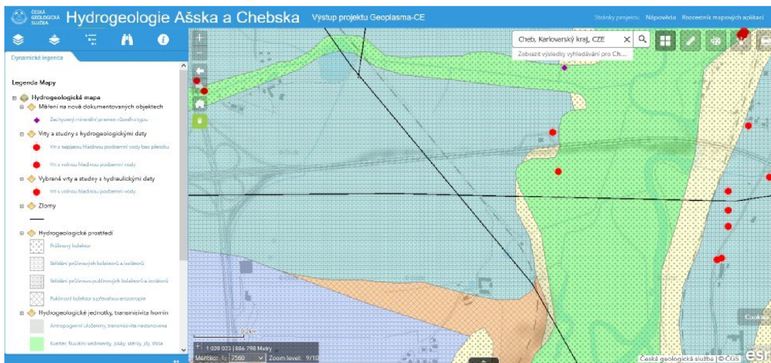
Obr. 22: Hydrogeologická mapka k. ú. Cheb (ČGS, © 2023)
