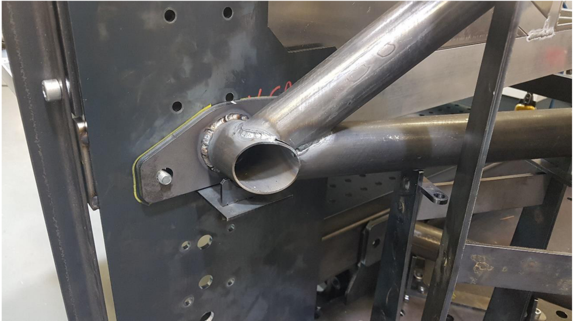
Obrázek 5: Detailní pohled na spoj hlavního rámu se spodním rohem E-boxu
