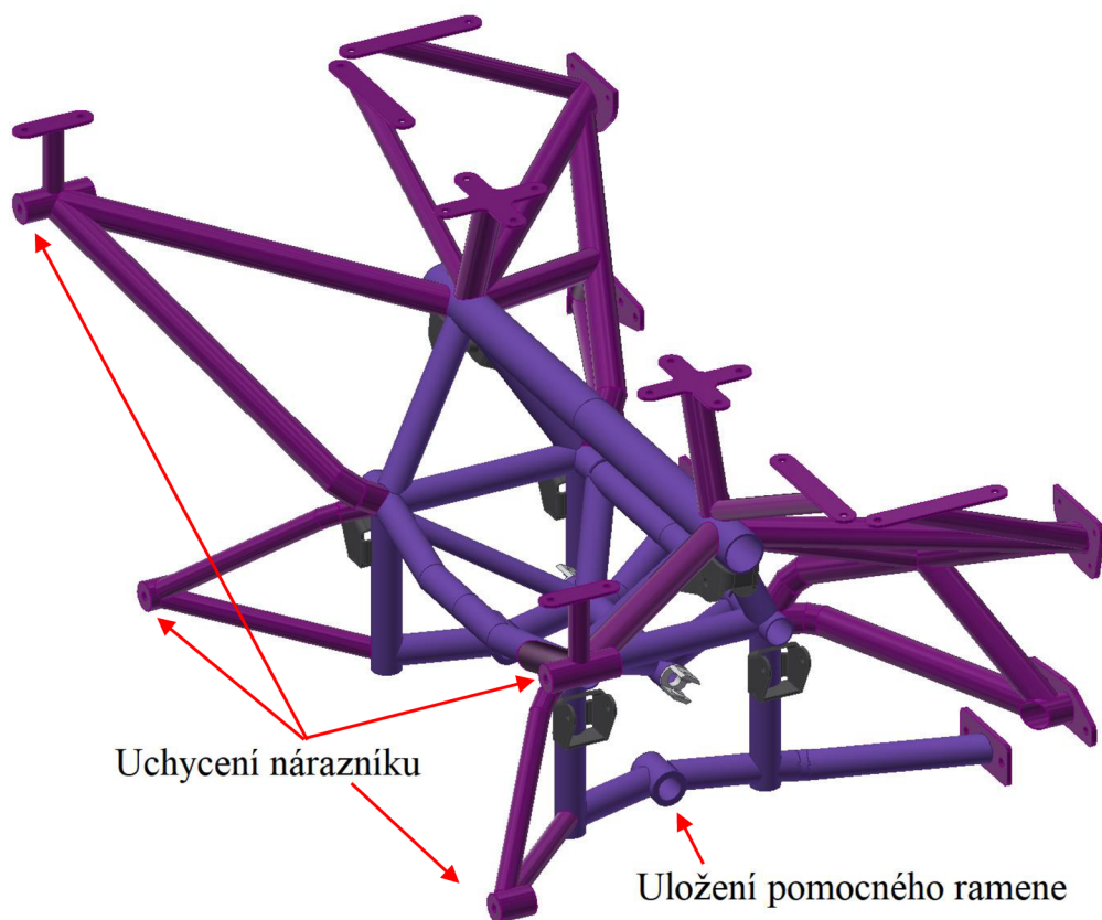
Obrázek 24: ISO pohled na 3D model hlavního rámu
