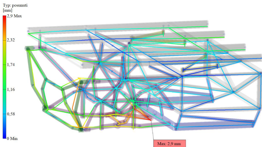
Obrázek 50: Výsledky simulace, posunutí – stav 4
