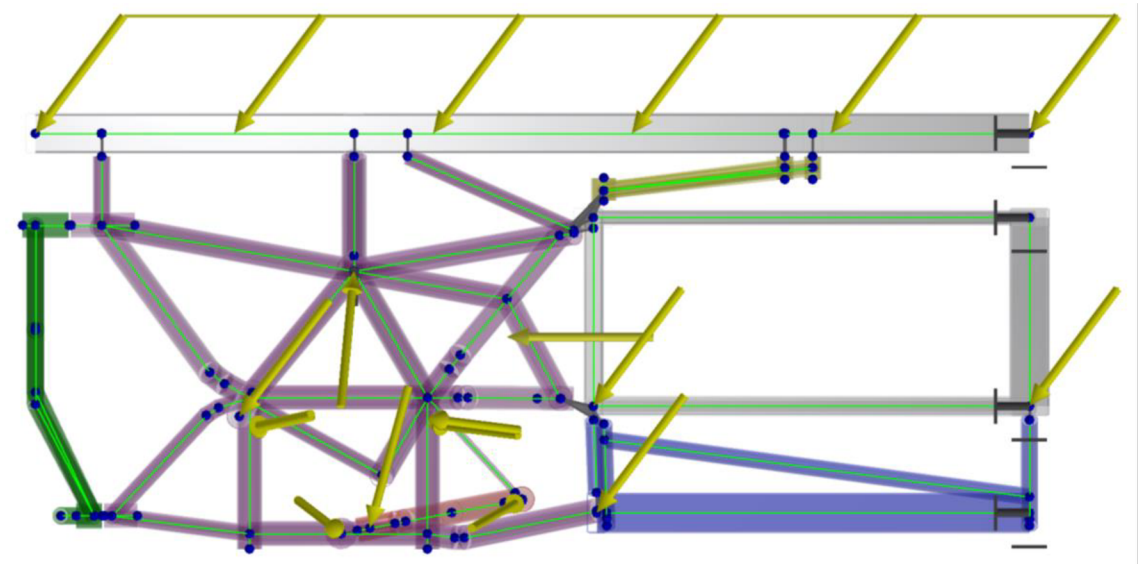
Obrázek 43: Zadané okrajové podmínky, boční pohled – stav 2
