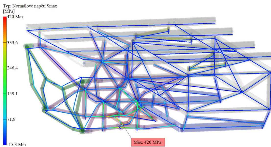
Obrázek 51: Výsledky simulace, napětí S_{max} – stav 4
