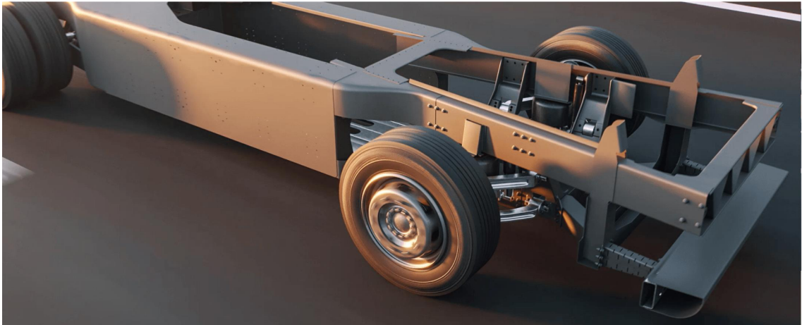
Obrázek 10: Podvozek modulární plošiny společnosti Gaussin [21]
