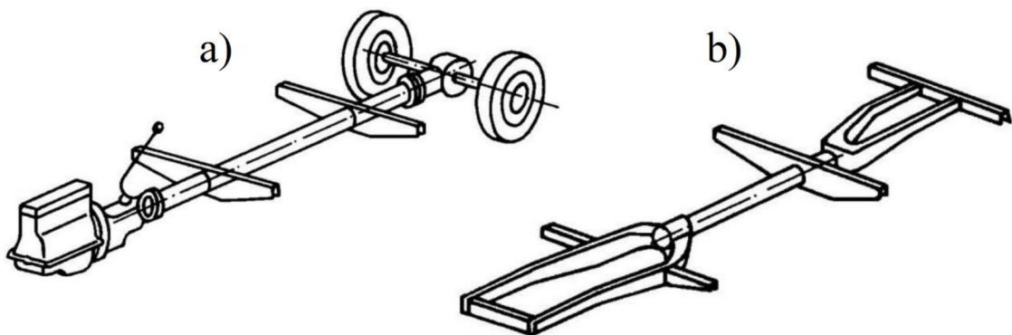
Obrázek 17: a) páteřový rám b) páteřový rám vidlicový
