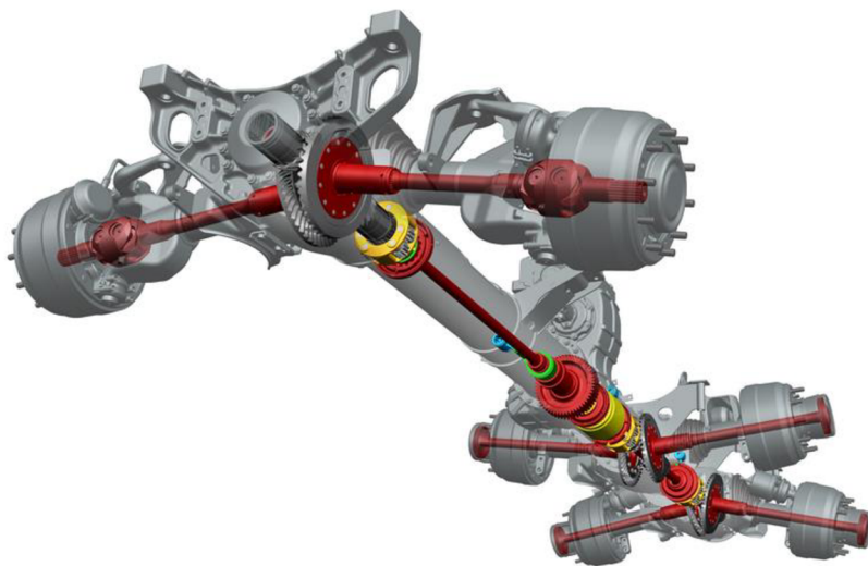
Obrázek 18: 3D model páteřového rámu vozidla od firmy Tatra [30]
