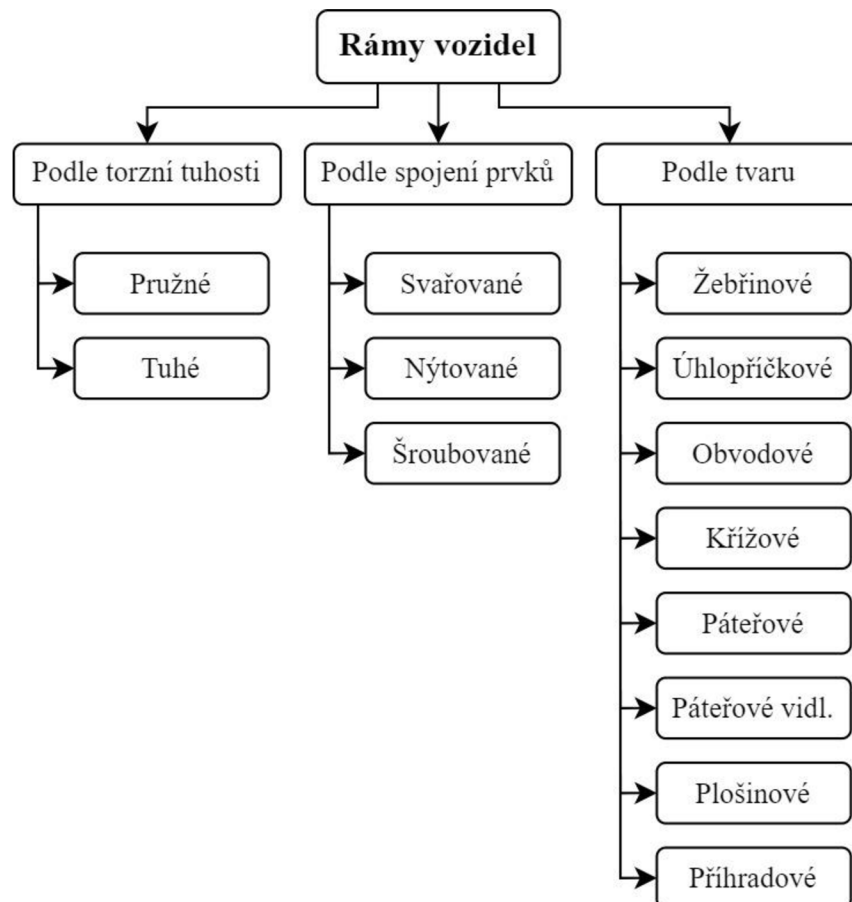
Obrázek 12: Grafické schéma rozdělení rámu vozidel [22]
