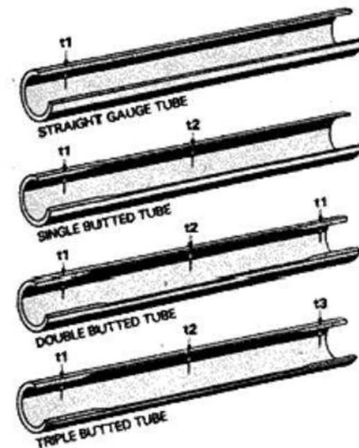
Obrázek 9.2: Zeslabování trubek – shora: nezeslabovaná, jednou zeslabovaná, dvakrát zeslabovaná a tříkrát zeslabovaná trubka [71]
