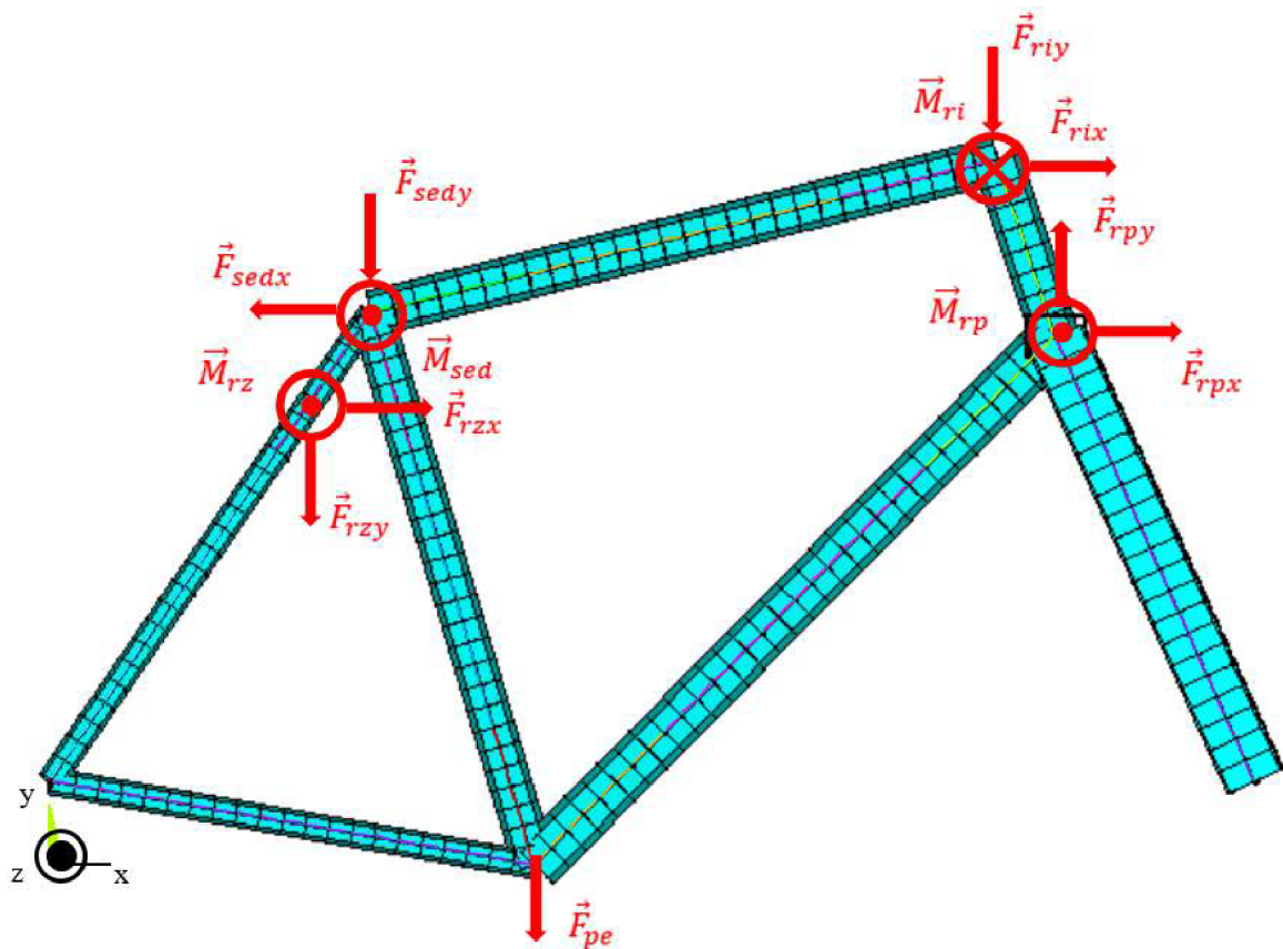
Obrázek 9.6: Silové působení na model pro ráfkové brzdy
