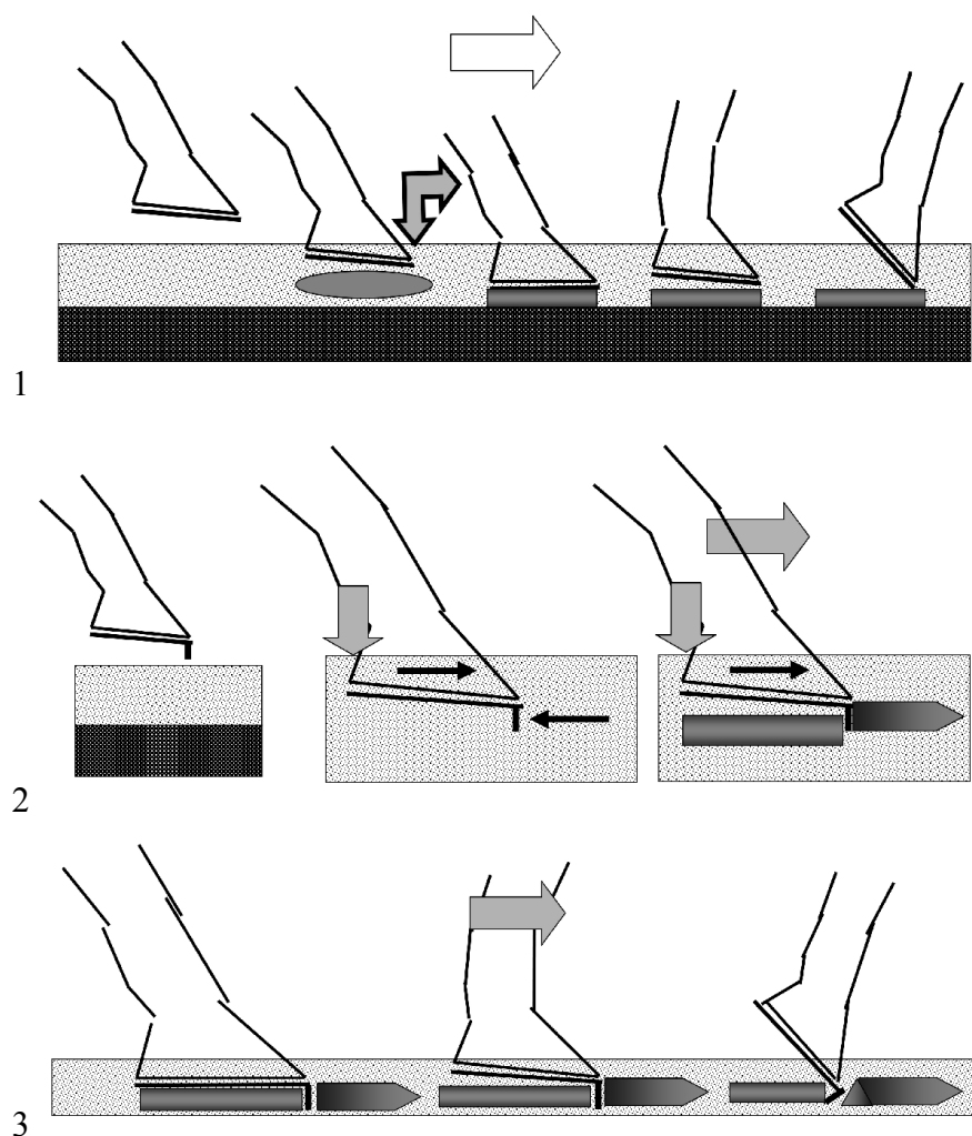
Obr.33: Porovnání dopadu kopyta s klasickou dostihovou podkovou (1) a s podkovou se zvýšeným okrajem („toe grab“; 2, 3) (GILLETTE & PETERSON, 2011)
