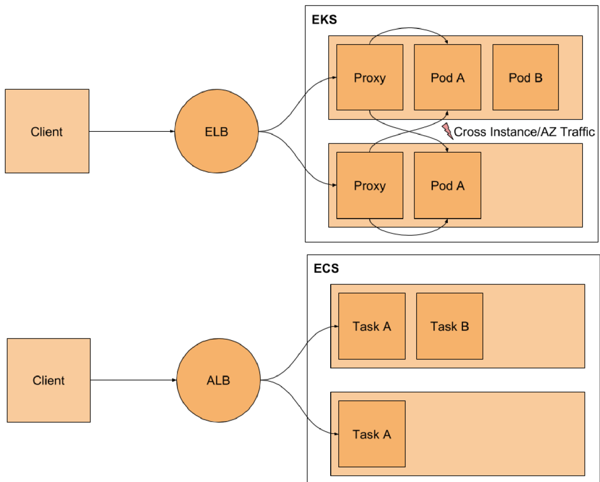
Obrázek č. 6. – porovnání architektur služeb EKS a ECS [44]
