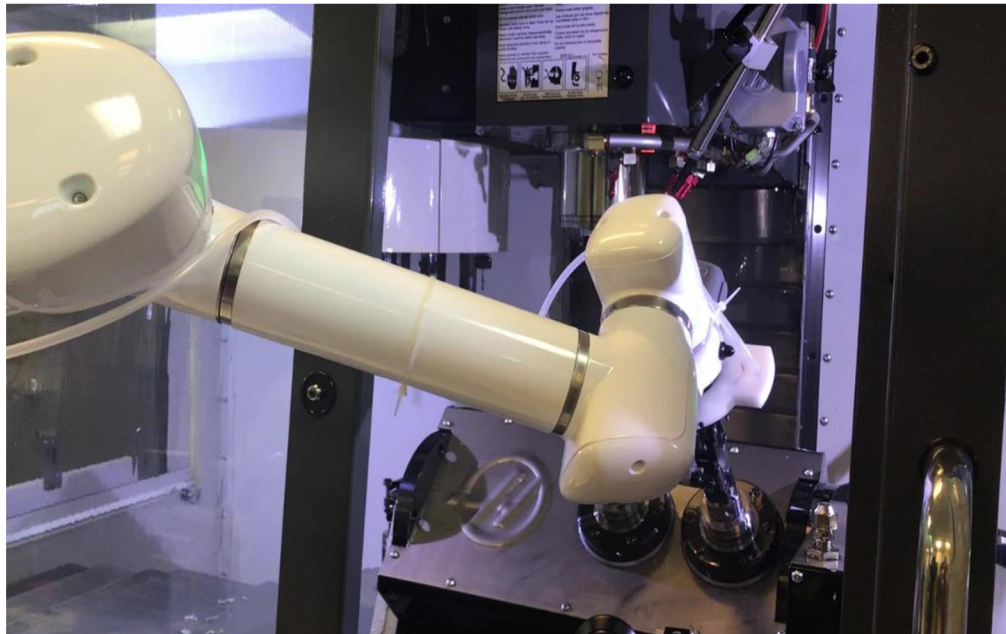
Obrázek 2.4: Obsluha CNC pomocí kobota [7]
