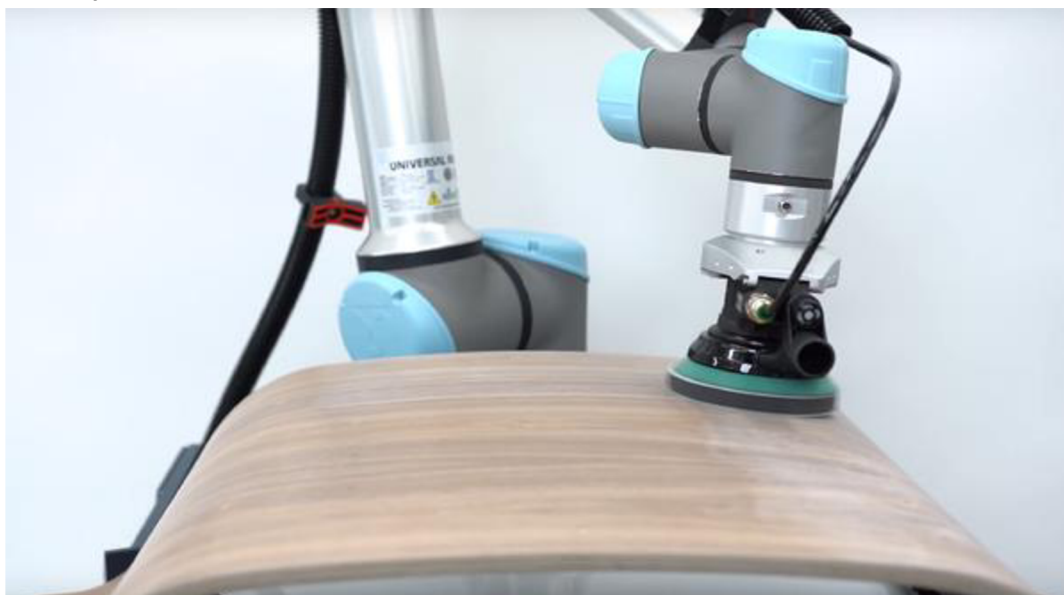
Obrázek 2.5: Broušení pomocí kobota [8]
