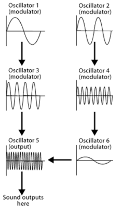
Obr. 2.2 FM syntéza [1]
