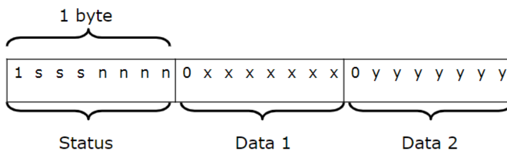
Obr. 2.7 Formát správy MIDI [6]
