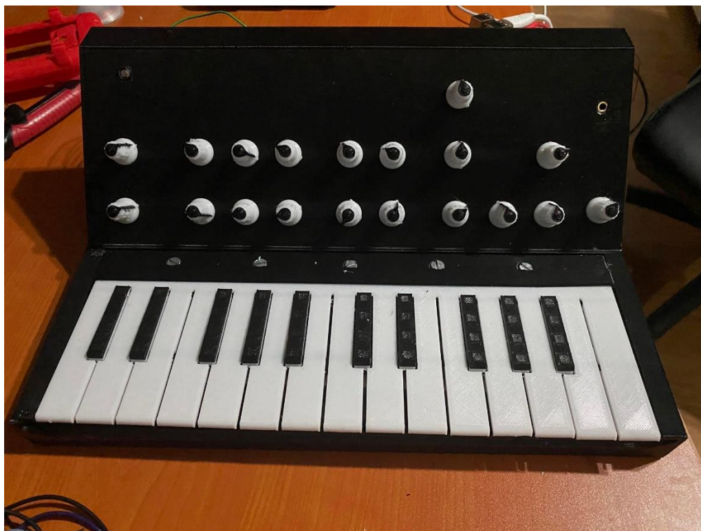
Obr. 4.1 Finálny výrobok
