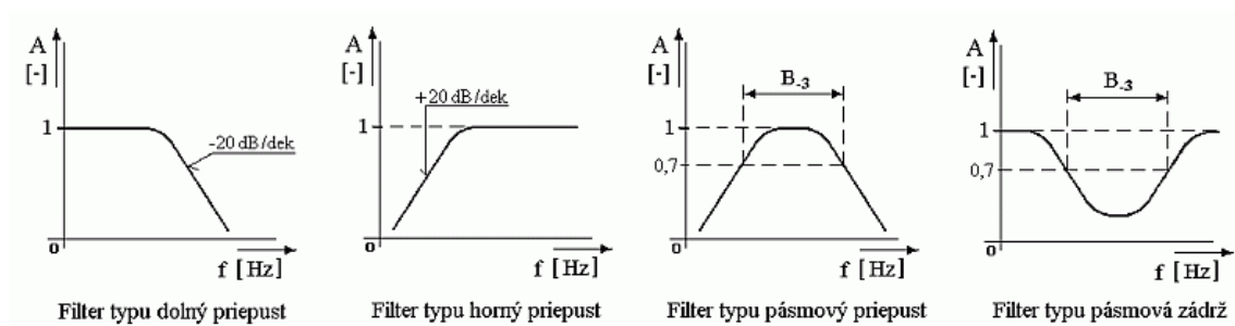
Obr. 2.3 Typy filtrov [3]
