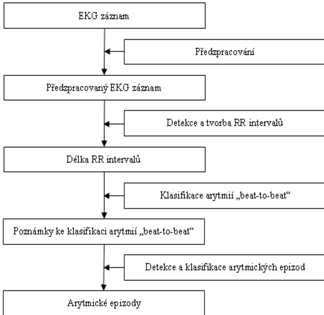
Obr. 4.12 Schéma užívaného detektoru a klasifikátoru arytmií
