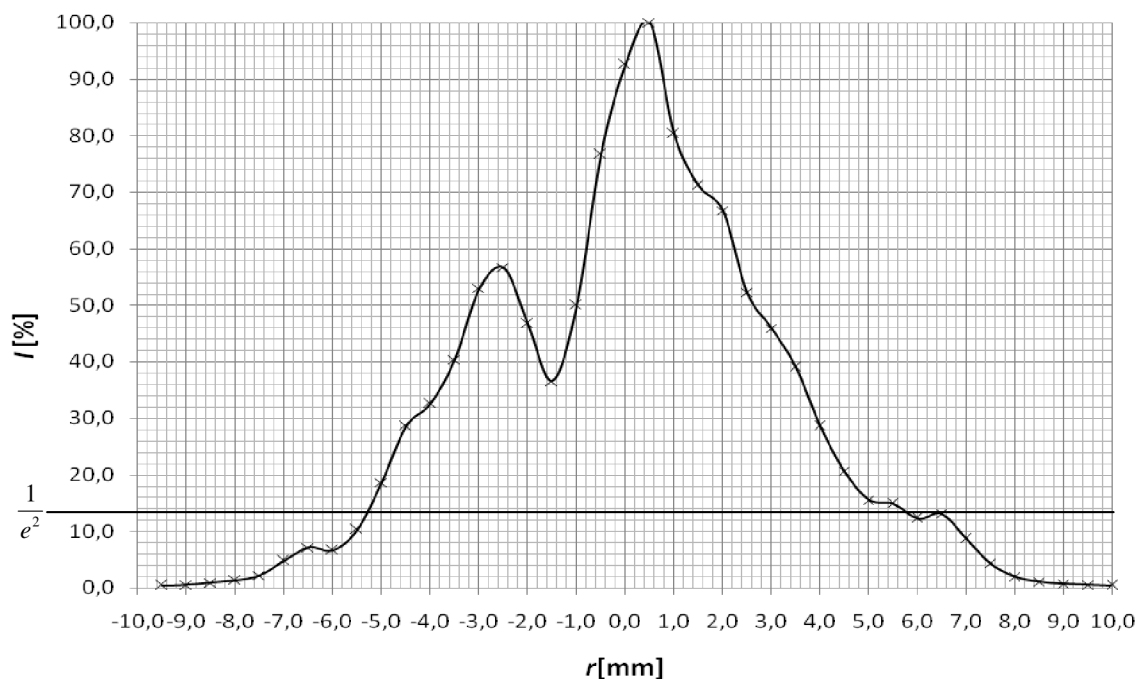
Obr.č.35: Rozložení optické intenzity vysílaného svazku s využitím MM vlákna (50/125) ve vzdálenosti z_l = 180 mm
