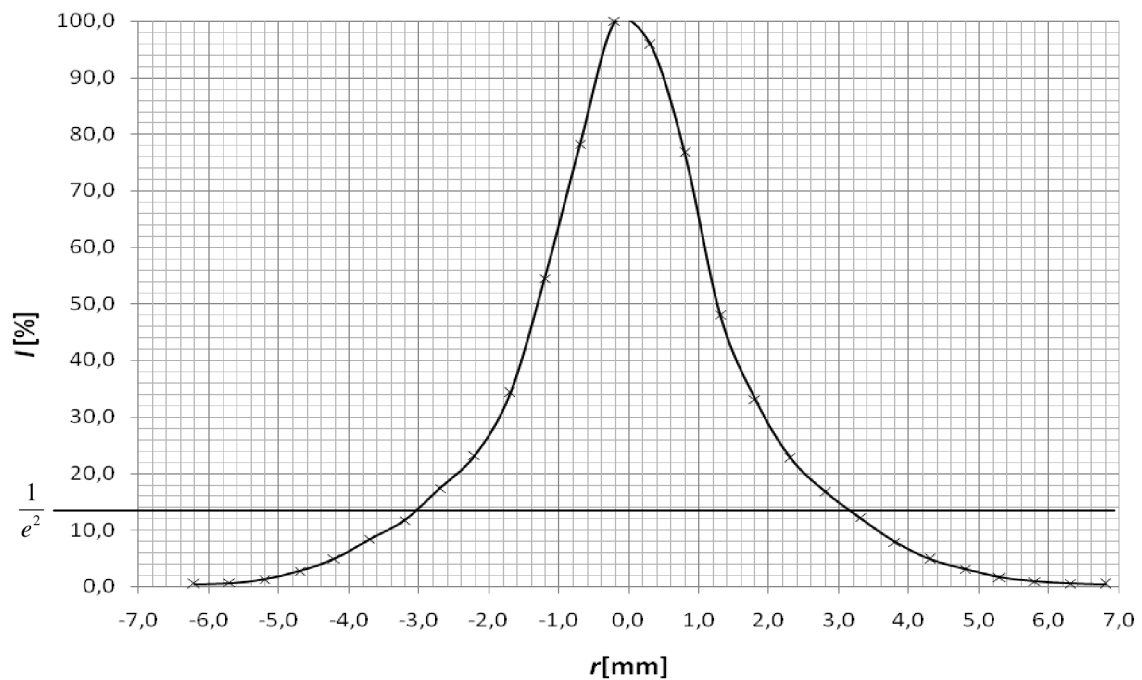
Obr.č.33: Rozložení optické intenzity vysílaného svazku s využitím SM vlákna (9/125) ve vzdálenosti z_l = 180 mm
