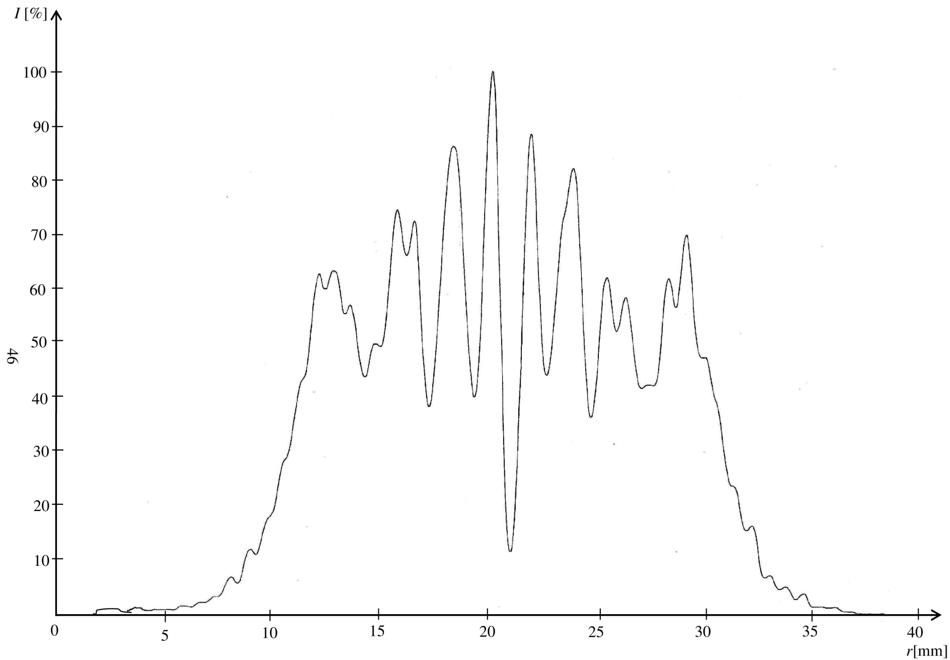
Obr.24: Příklad rozložení optické intenzity v difrakčním obrazci ( D_{ST} = 5 mm, z = 3 m, D_{ST}/2w_{TXA} = 0,42 )
