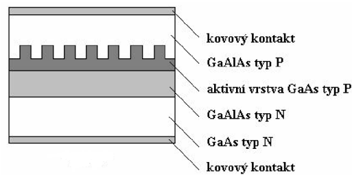
Obr.19: Laser s rozloženou zpětnou vazbou – DBFL (podle [7])
