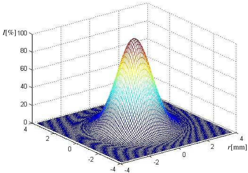
Obr.20: 3D zobrazení vyzařovací charakteristiky SM vlákna (9/125) ve vzdálenosti l = 40 mm
