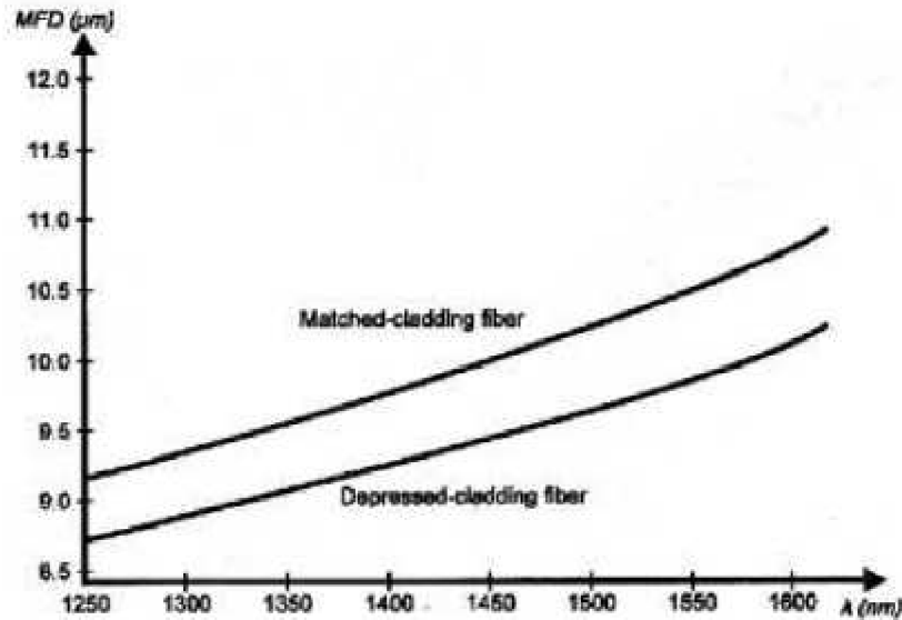
Obr.12: Závislost modového pole MFD na vlnové délce (podle [1])
