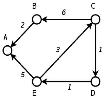
Obr. 4 – Hranově ohodnocený graf
