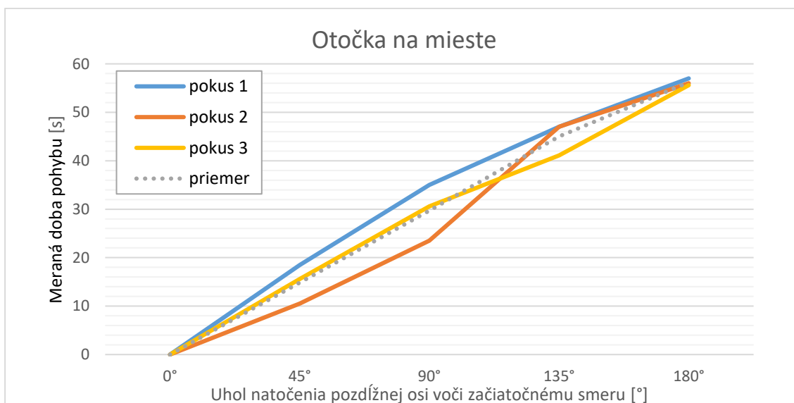
Obr. 64: Graf uhlovej rýchlosti počas pribehu otáčania sa o 180°
