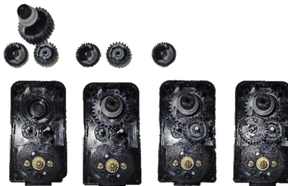
Obr. 25: Prevedovka aktuátora AX-12
