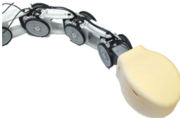
Obr. 67: Detail planárneho robotického hada
