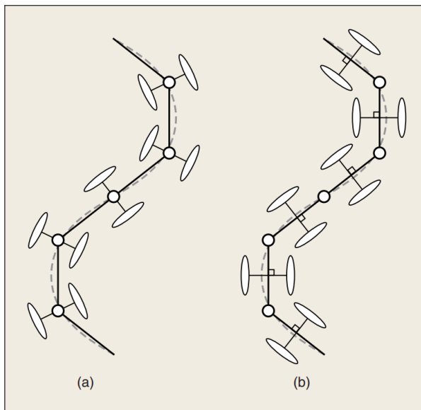
Obr. 15: Rozdiel polohy a uloženia kolies medzi robotmi ACM-III (a) a ACM-R3 (b) [8]
