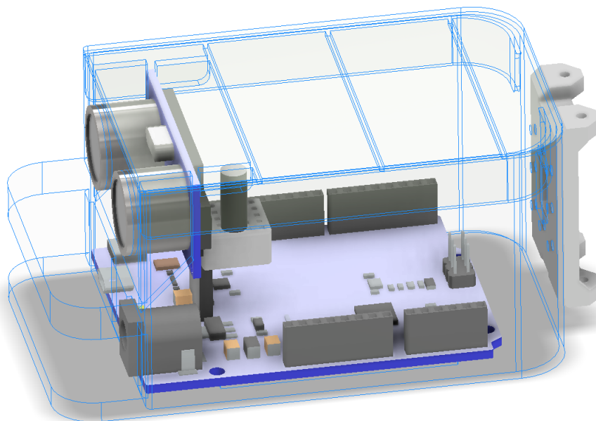
Obr. 44: Vnútorné rozloženie komponentov
