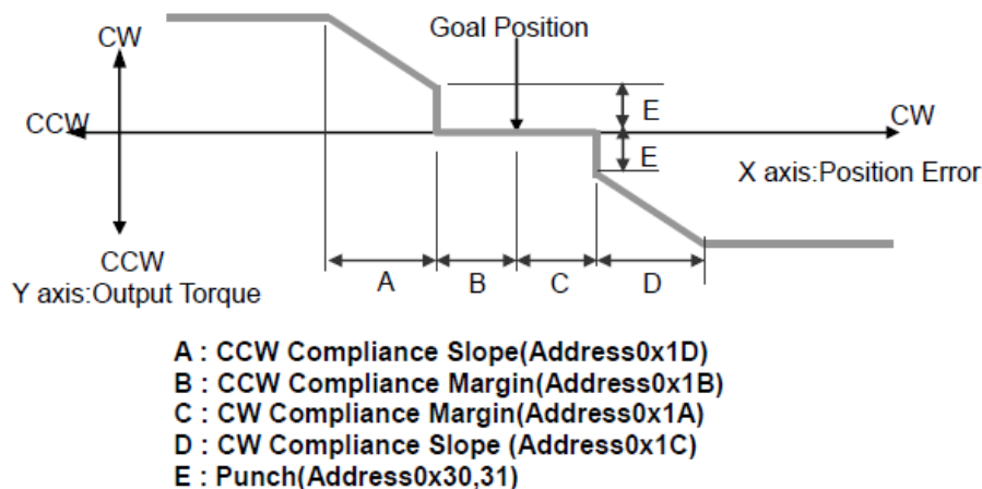
Obr. 29: Spätaná väzba aktuátora Dynamixel AX-12 [12]
