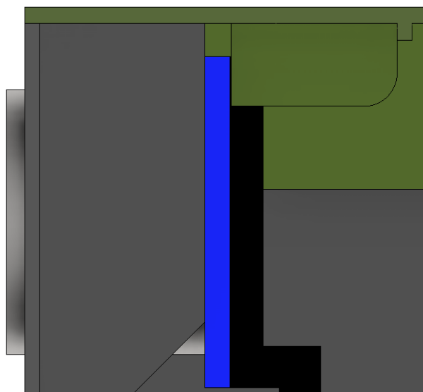
Obr. 47: Bočný prierez hlavou zobrazujúci uchytenie dosky plošných spojov senzora
