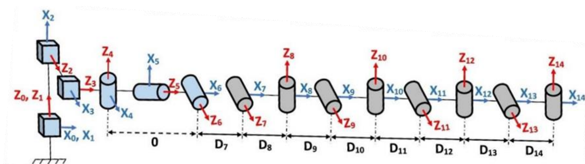
Obr. 36: Kinematická štruktúra [14]
