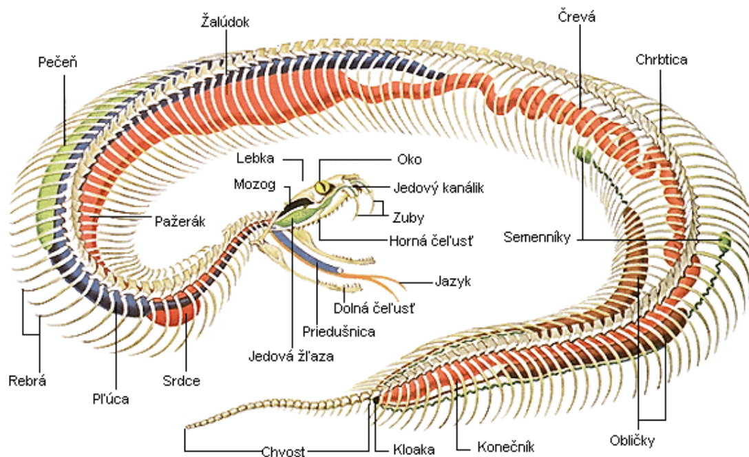
Obr. 4: Anatómia hada [6]
