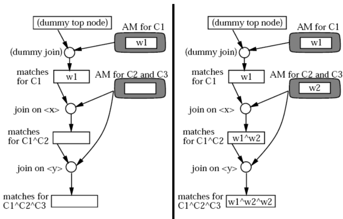
Obrázek 2. Spojovací uzly mezi jednotlivými podmínkami inferenčního pravidla[1]
