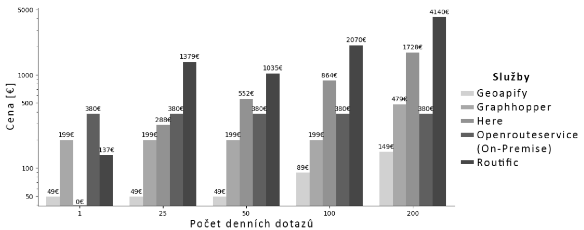
Obrázek B.4: 10 aut a 15 lokací v dotazu ( request )
