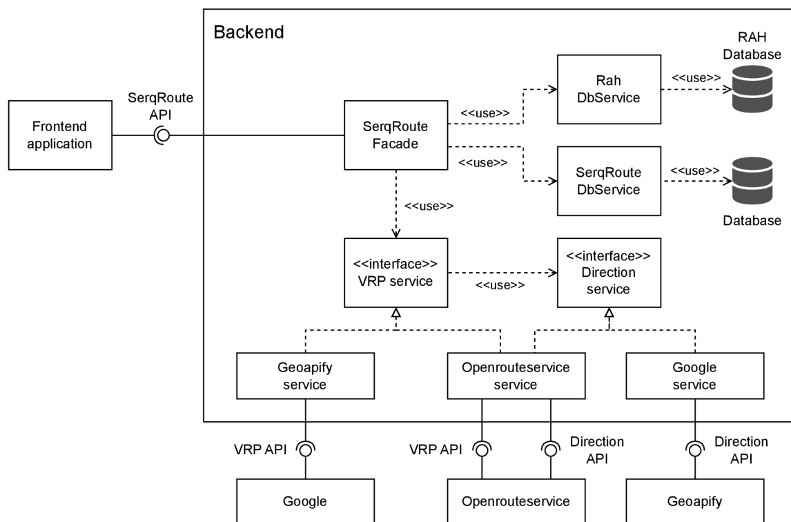
Obrázek 6.1: Návrh architektury řešení.
