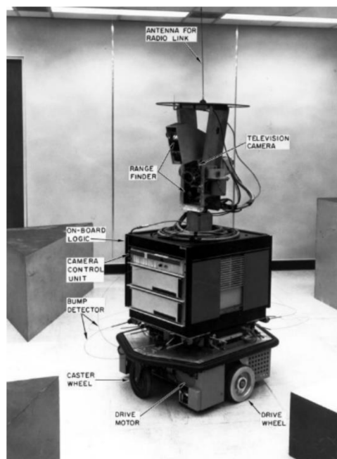
Obrázek 7 - Robot Shakey
