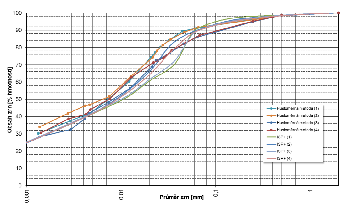
Obr. 13: Výsledné čáry zrnitosti pro vzorek hlinité půdy – porovnání hustoměrné metody a metody ISP+.
