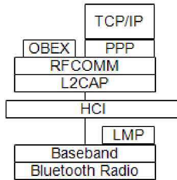
Obrázek 3.1: Vrstvy protokolů
