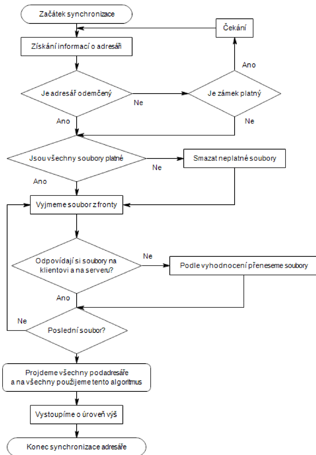
Obrázek A.2: Diagram algoritmu synchronizace
