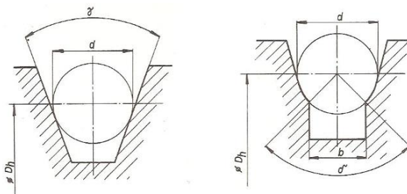
Obr. 9 Klínová drážka [5] Obr. 10 Polokruhová drážka se zářezem [5]
