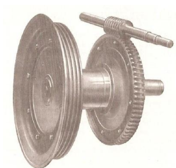
Obr. 6 Šnekový převod (šnek a šnekové kolo) [4]
