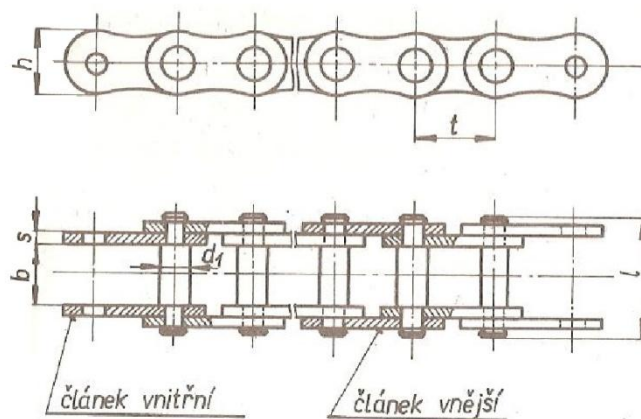
Obr. 14 Gallův řetěz [1]
