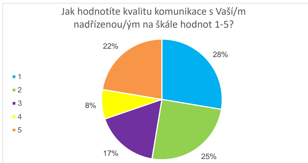
Obrázek 16: Graf znázornění kvality komunikace od nadřízené/ho
