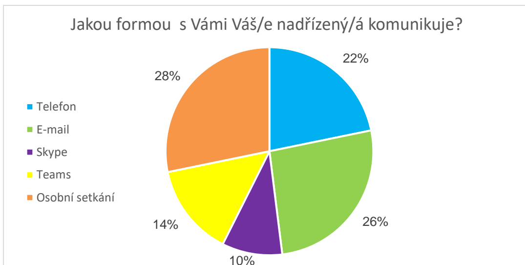
Obrázek 17: Graf formy komunikace s nadřízenou/ým
