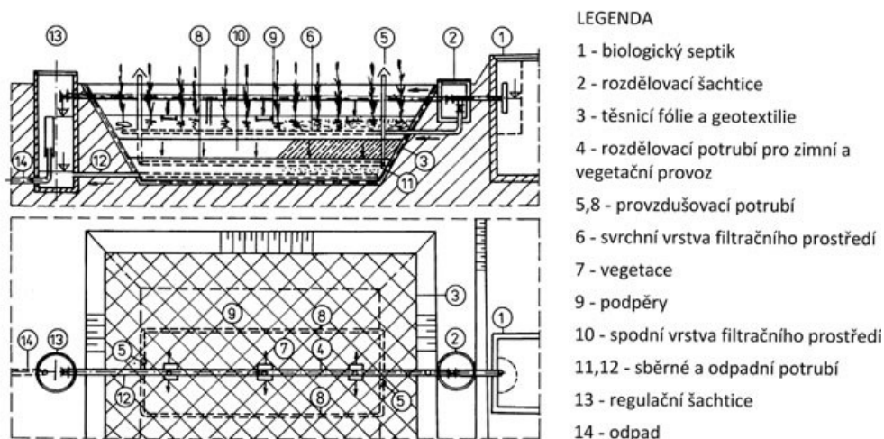
Obrázek 16 Vertikální filtr (Šálek a kol., 2013)
