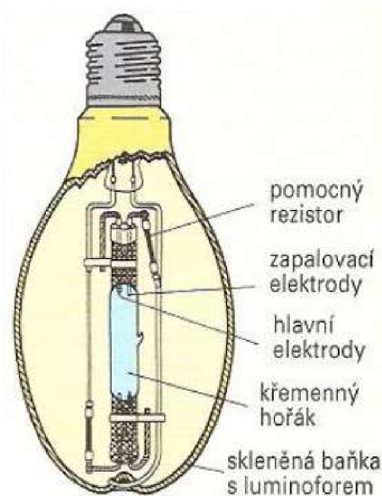
Obrázek 2.2 Konstrukce vysokotlakého výbojového zdroje[6].
