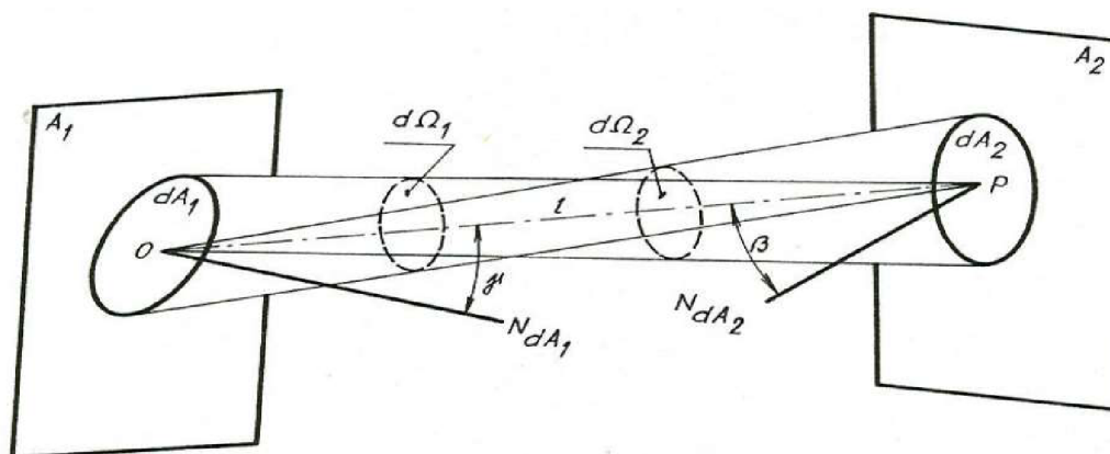
Obrázek 1.3 Vymezení svazků paprsků mezi plochami [3].
