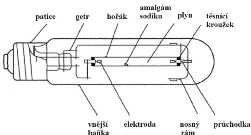
Obrázek 2.4 Konstrukce vysokotlaké sodíkové výbojky [7].
