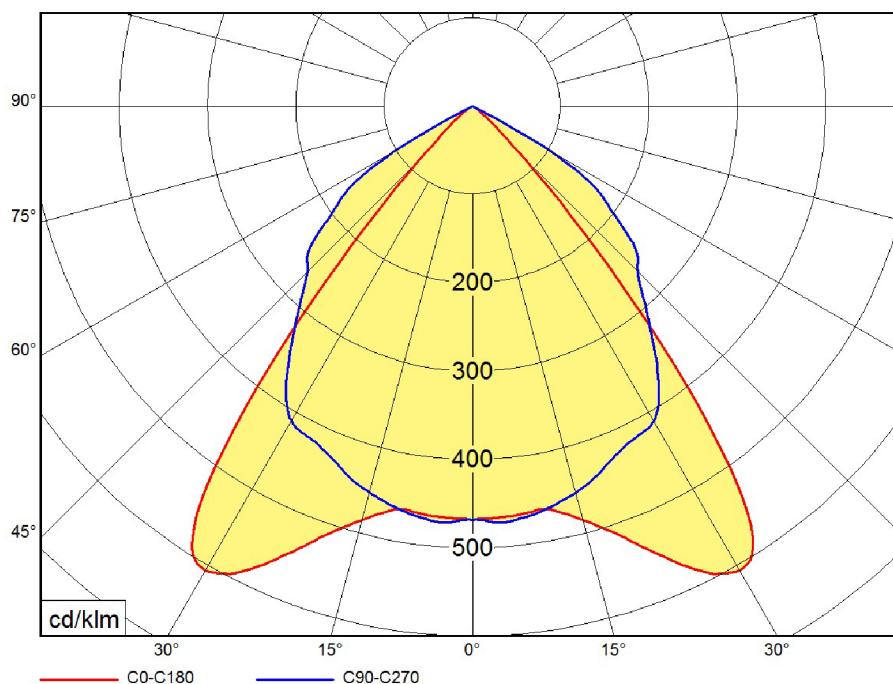
Obrázek 3.1 Křivka svítivosti panelového svítlidla s mřížovou clonou [9].
