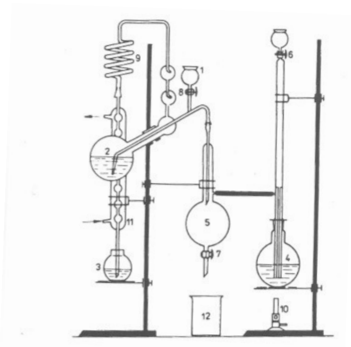
Obrázok 3: Parnas-Wagnerova aparátúra [35]
