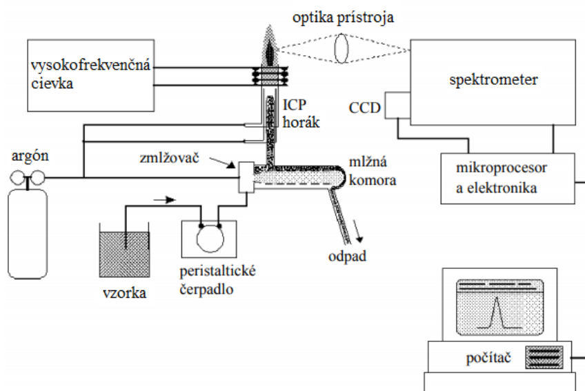
Obrázok 7: Schéma ICP-OES [43]
