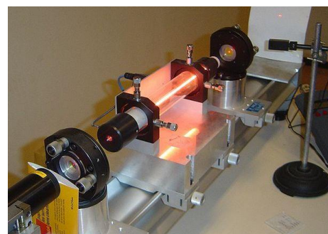
Obrázek 7.2: Helium-Neonový laser [11]
