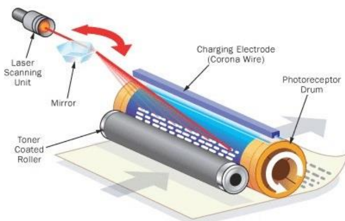
Obrázek 8.9: Princip laserové tiskárny [26]
