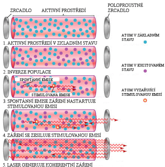
Obrázek 6.4: Princip laseru [29]
