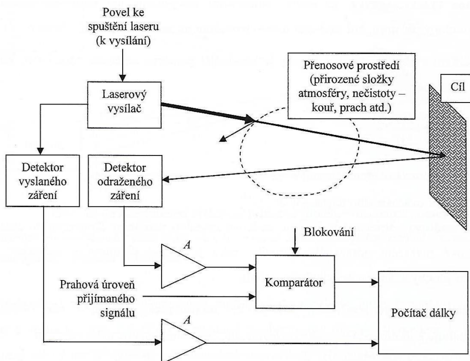
Obrázek 10.1: Principiální blokové schéma laserového dálkoměru [33]
