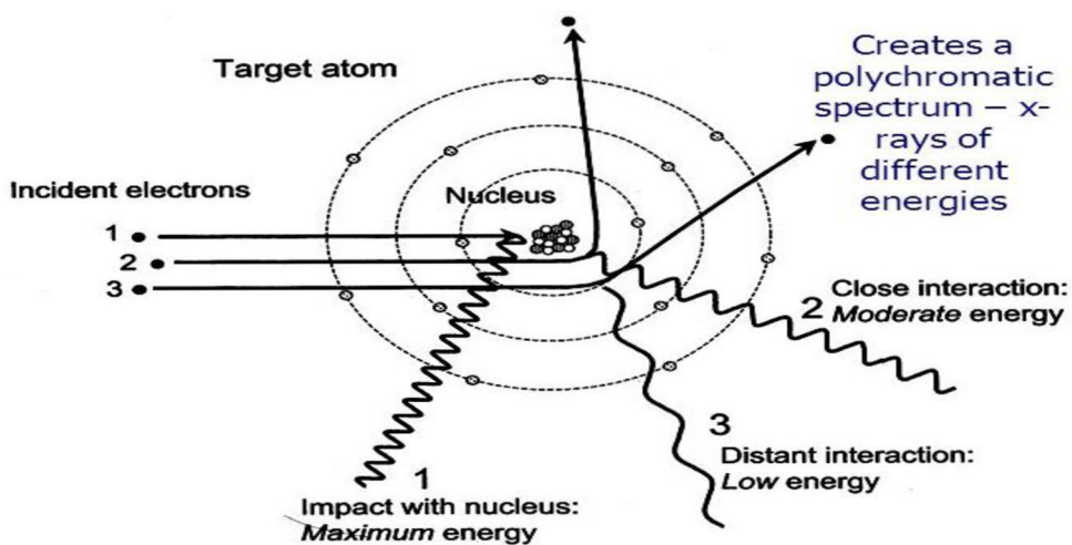
Obrázek 7: X-ray fotony
