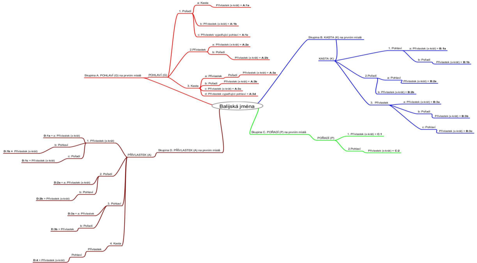
Obrázek č. 1 - Myšlenková mapa vysvětlující rozřazení skupin podle složení balijských jmen
