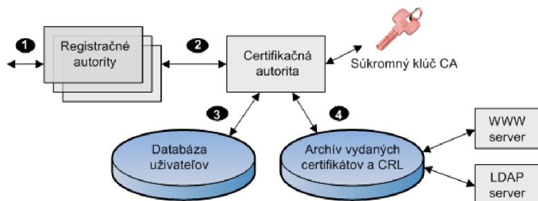
Obr.4.2: Štruktúra certifikačnej autority.
