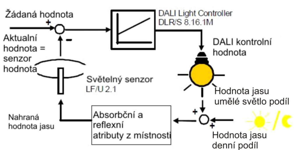
Obr. 7-15 Laboratorní návod 2 – Princip zastoupení stálých světel
