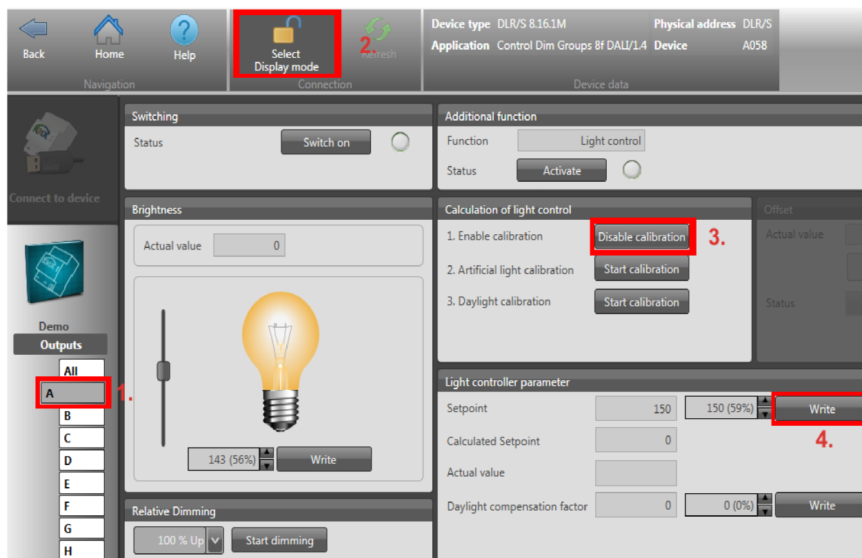
Obr. 7-20 Laboratorní návod 2 – Nastavení nástroje „i-bus tool“
