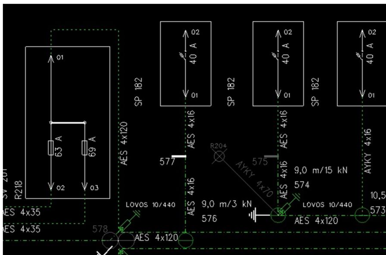
Obrázek 2: Jednopolové schéma v programu SPIDER-EN
