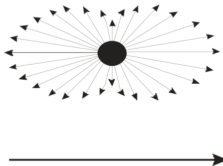
Obr. 2.3: Raylegův rozptyl (šipka určuje směr odkud přichází rozptylové záření) [14]
