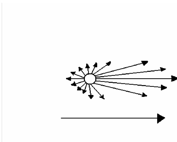
Obr.2.4: Mieův rozptyl [14]
