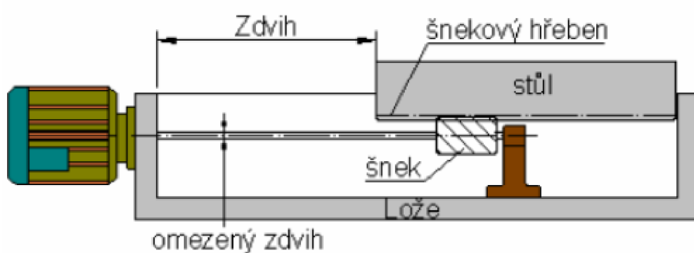
Obr. 6 Schéma šneku a šnekového hřebenu [23]
