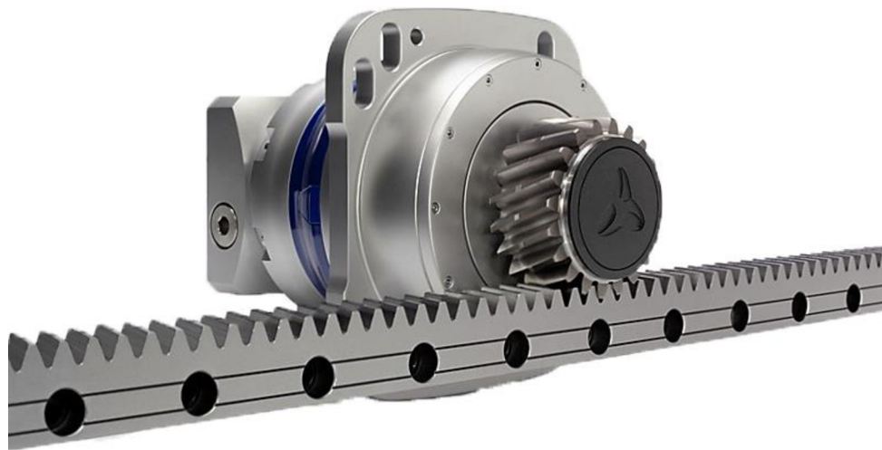
Obr. 5 Pastorek a hřeben [15]
