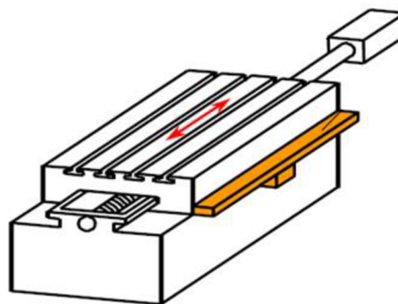
Obr. 12 Přímé odměřování [18]
