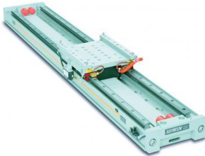
Obr. 1 Lineární osa s lineárním pohonem [13]
