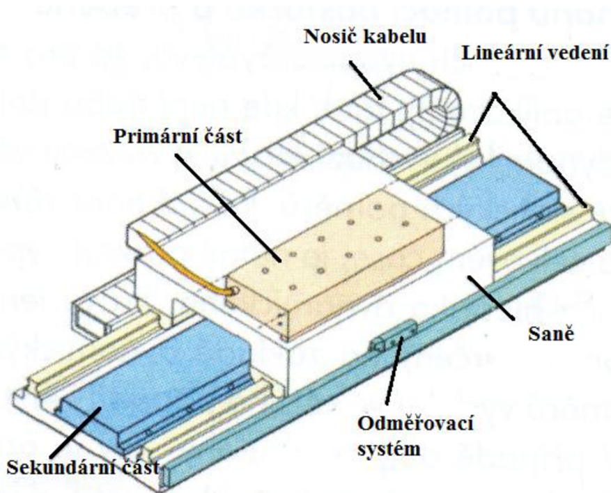
Obr. 8 Lineární motor [16]
