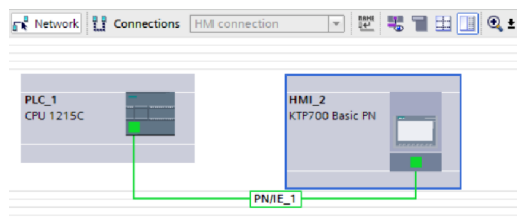
Obrázek 10.1: Propojení HMI k PLC v TIA portal
