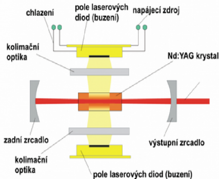
Obrázek 2.3: Boční čerpání [12]
