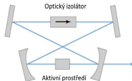
Obrázek 2.9: Kruhový rezonátor [14]
