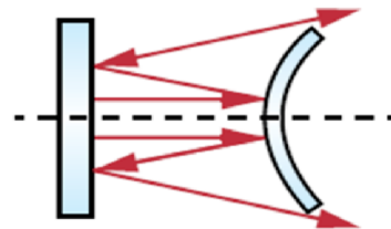
Obrázek 2.7: Nestabilní rezonátor [16]
