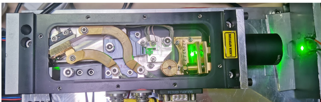
Obrázek 3.2: Vnitřní uspořádání laseru JenLas D2.3
