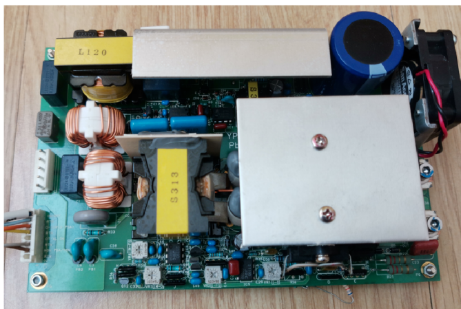
Obrázek 3.6: Laserový zdroj
