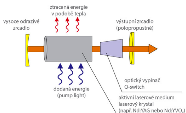
Obrázek 2.5: Schéma pevnolátkového laseru s rezonátorem [15]
