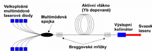
Obrázek 2.11: Princip vláknového laseru [12]
