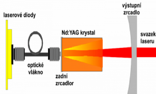
Obrázek 2.4: Zadní čerpání [12]
