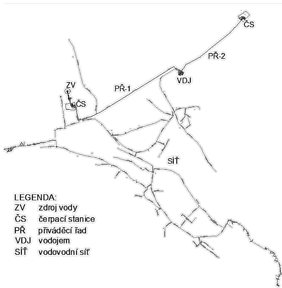
Obrázek 5.11 Schéma hodnocené vodovodní sítě TP2-BOR
