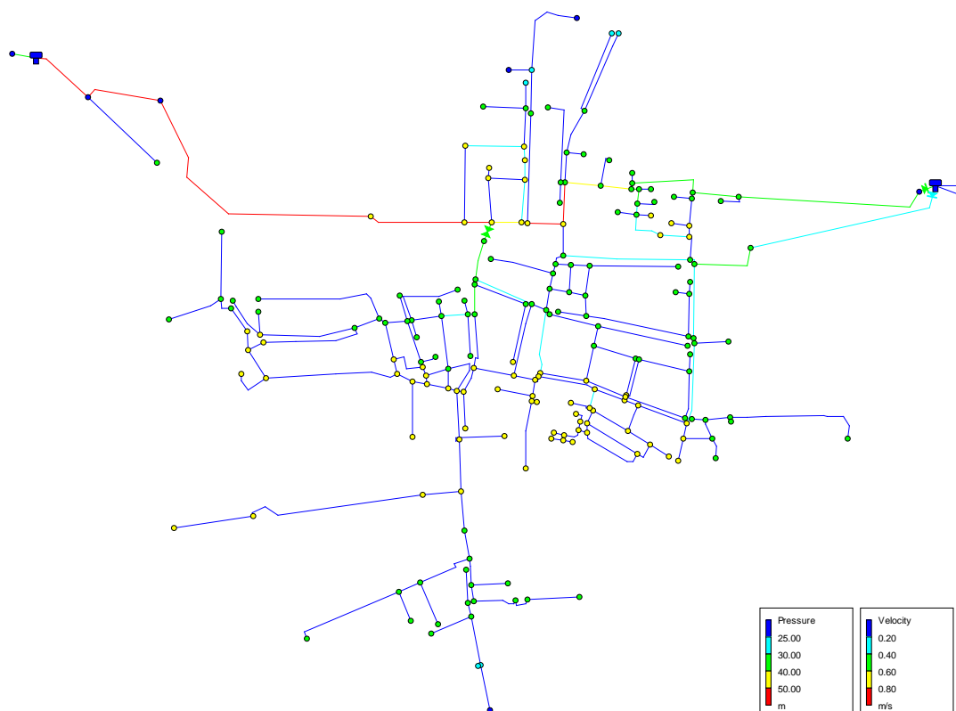
Obrázek 5.10 Schéma hodnocené vodovodní sítě TP1-SL
