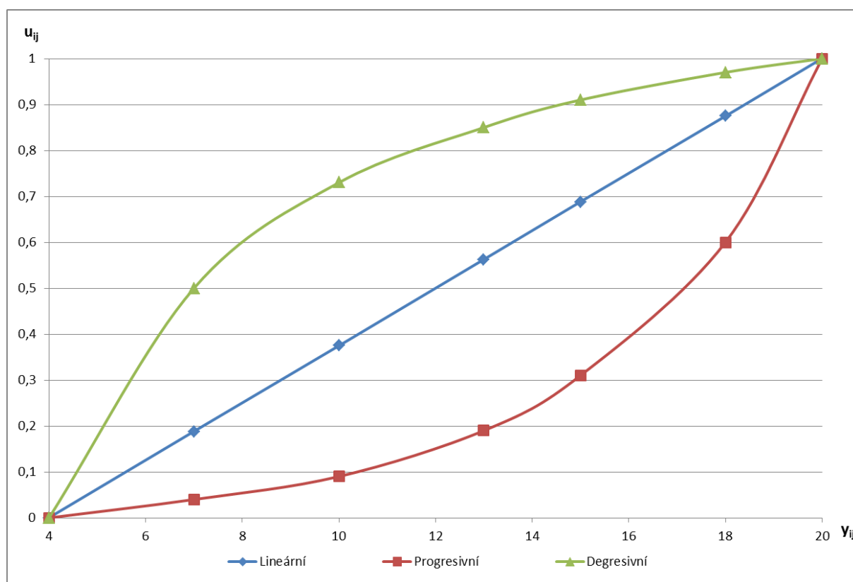
Obrázek 3.9 Příklad lineární, progresivní a degresivní dílčí funkce užitku [31]
