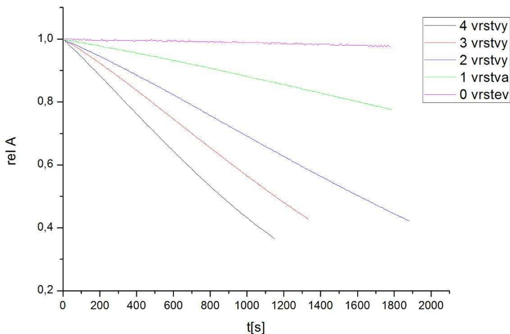
Graf 3: Závislost zprůměrovaných relativních dat absorpance na čase ozařování
