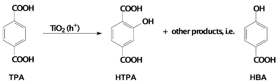
Obrázek 14: Fotokatalytická oxidace TPA
