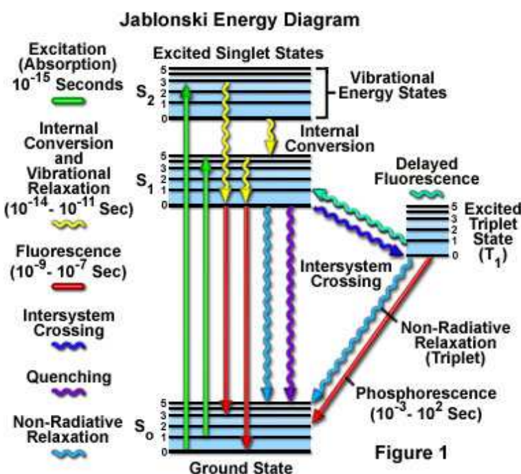
Obrázek 21: Jablonského diagram 35
