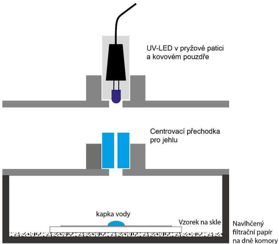
Obrázek 26: Schéma reaktoru pro měření kontaktního úhlu
