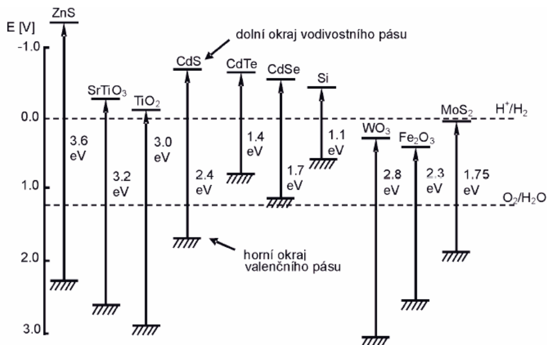
Obrázek 2: Poloha a šířka zakázaných pásů vybraných polovodičů 2
