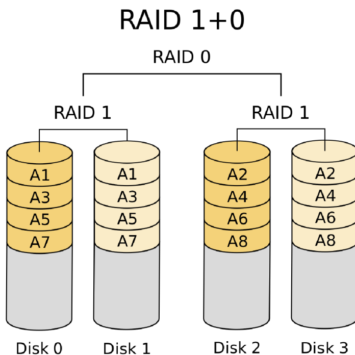
Obrázek 5 Schéma RAID 10
