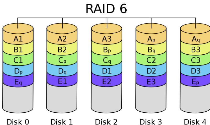
Obrázek 4 Schéma RAID 6
