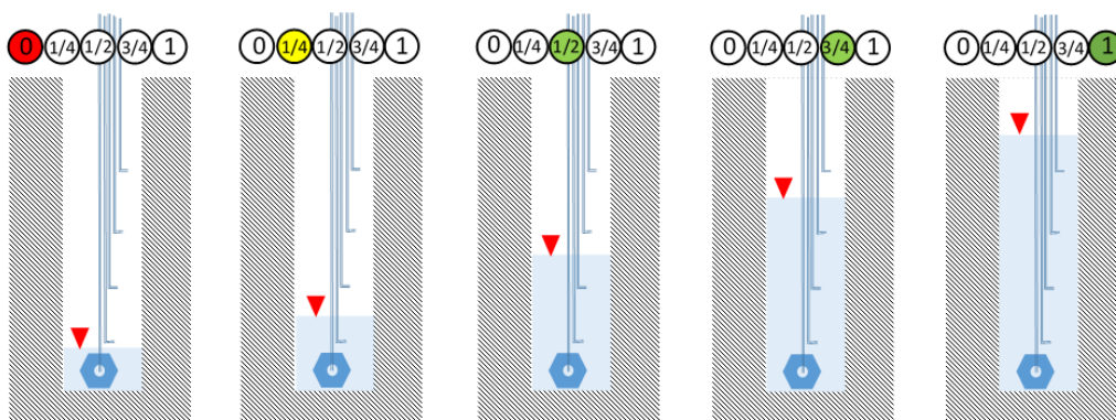
Obrázek 1.3 Princip funkce měření hladiny vodivostními hladinoměry [3]
