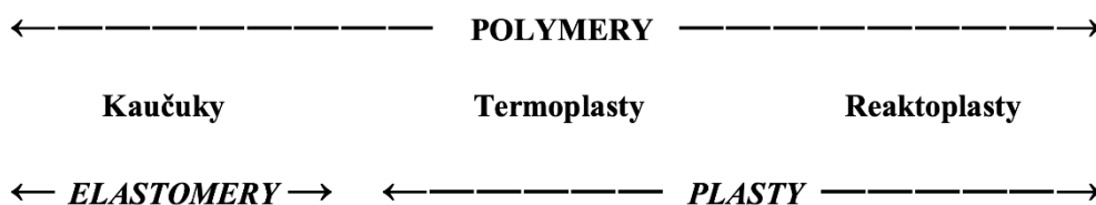
Obr. 2.1 Delenie polymérov [18].
