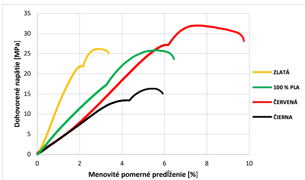
Obr. 4.10 Ťahový diagram.
