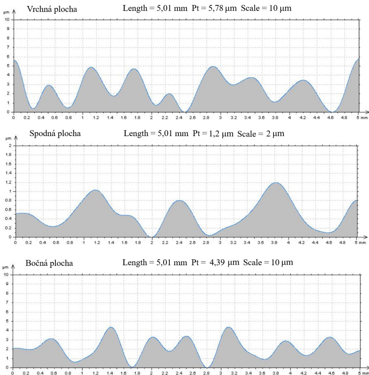
Obr. 4.25 Profily vlnitosti povrchu vzorky s červeným aditívom.
