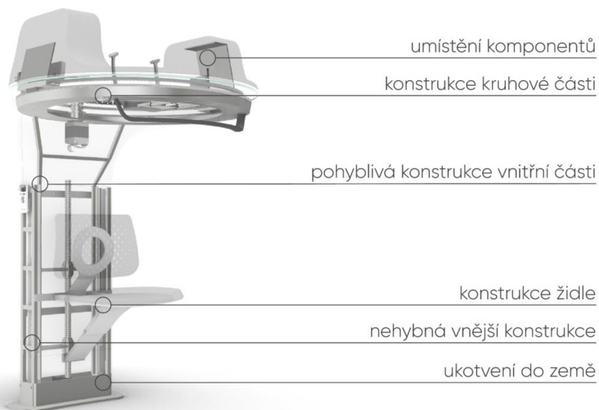
Obr. 6-7 Vnitřní konstrukce
