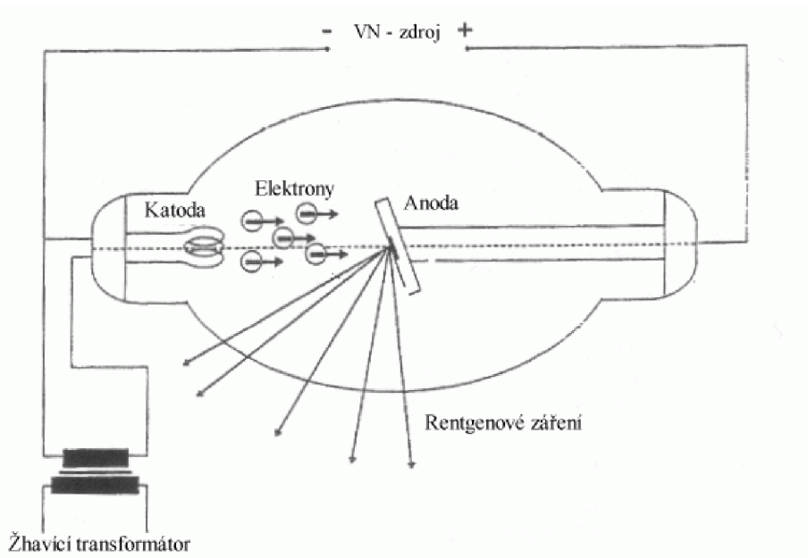
Obr. 2-17 Schéma rentgenky [24]
