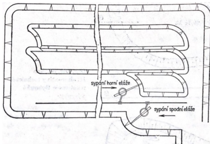
Obr. 13 Technologie bočního sypání pásovým zakládačem <Štýs a kol., 1981>
