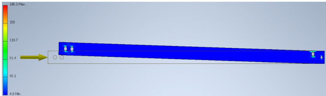
Obrázek 2.IV – Rozložení napětí v delším bočním nosníku v MPa
