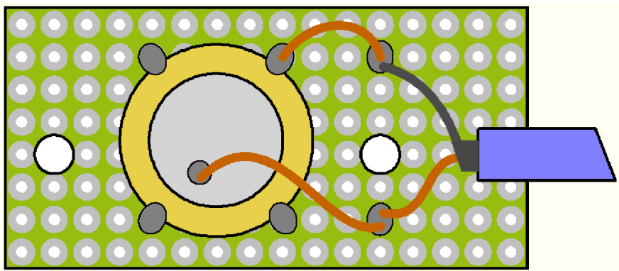
Obrázek 2.XVI – Měnič na zkušební desce
