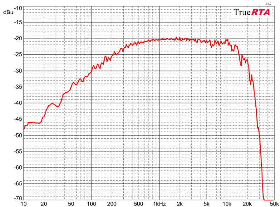
Obrázek 2.XXI – Kmitočtová charakteristika zesilovače pro plné zesílení
