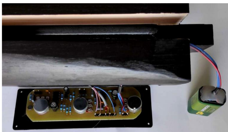
Obrázek 3.XVI – Ovládací panel před montáží
