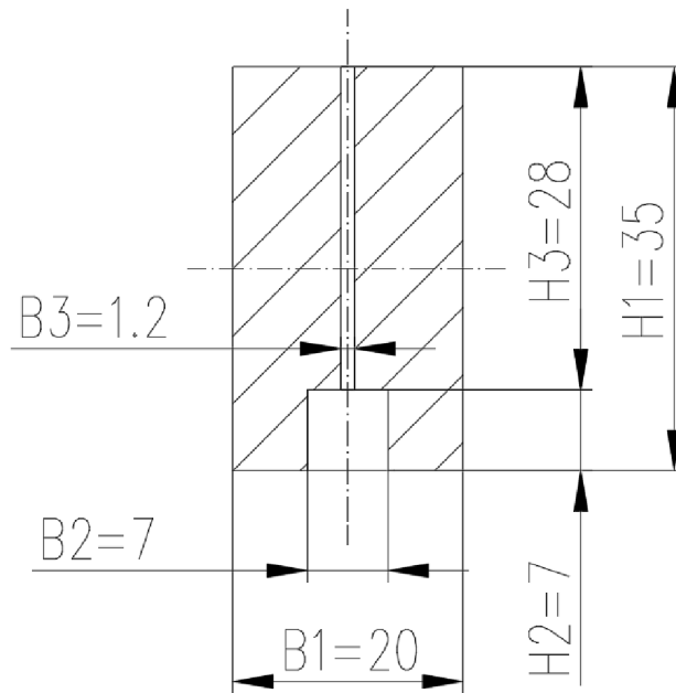
Obrázek 2.VII – zobrazení průřezu polotovaru [mm] [9]
