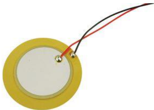
Obrázek 2.XV – Piezo snímač 15mm
