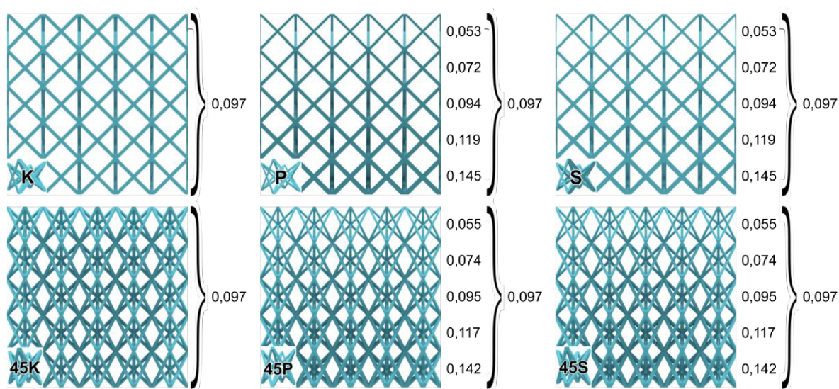
Obr. 4-4 Relativní hustoty struktur
