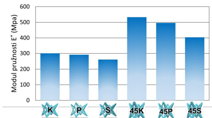
Obr. 5-9 Modul pružnosti struktur
