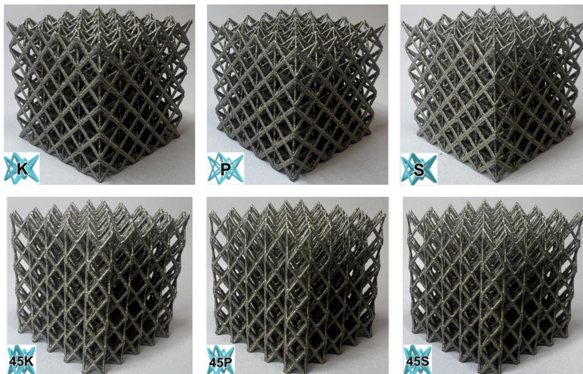
Obr. 5-1 Fotodokumentace struktur
