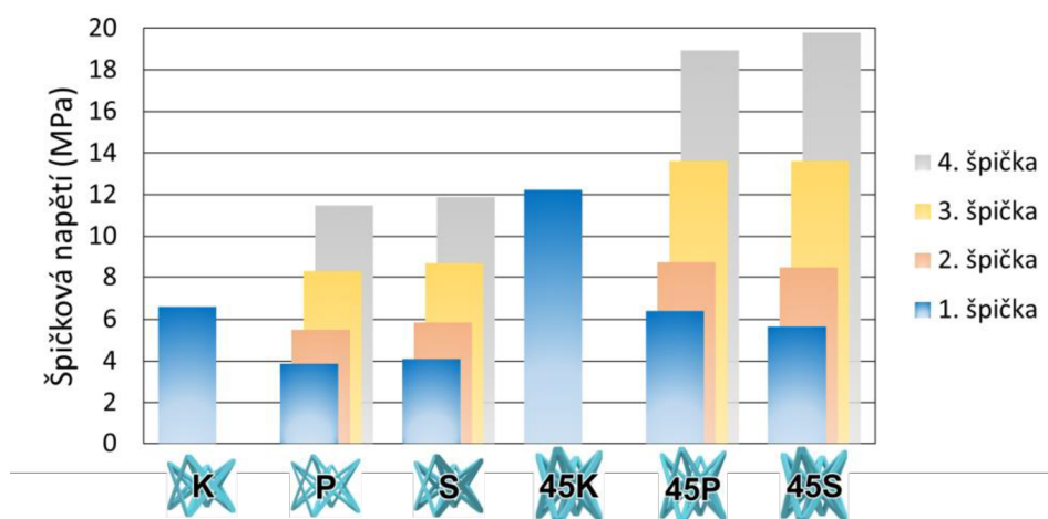
Obr. 5-8 Hodnoty dosažených špičkových napětí
