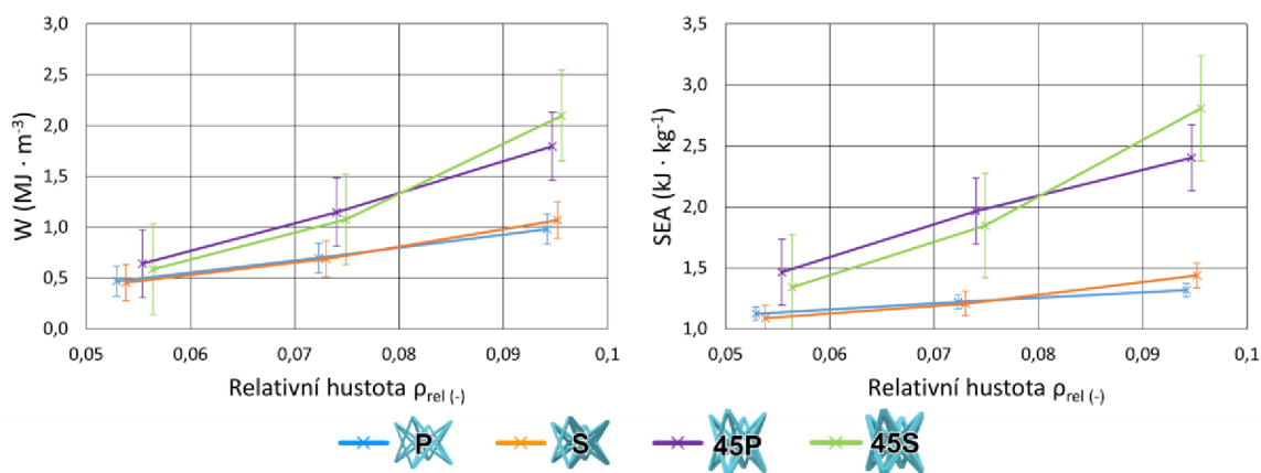
Obr. 5-14 Závislost absorbované energie na relativní hustotě
