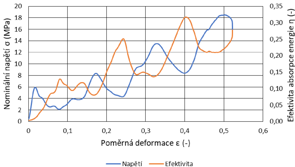
Obr. 5-11 Porovnání závislosti napětí a efektivity na poměrné deformaci (vzorek 45P4)
